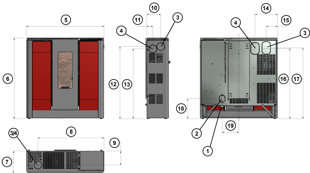
Fig. 13 - Dimensões gerais: Style
