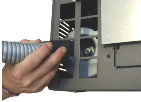
Fig. 49 - Limpeza do ventilador ambiente
