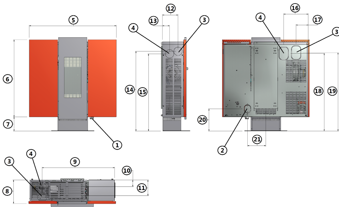
Fig. 12 - Dimensões gerais: Wall/Small
