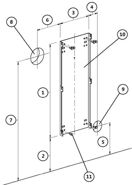
Fig. 16 - Fixação em parede não inflamável
