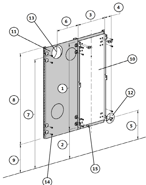
Fig. 17 - Fixação em parede não inflamável
