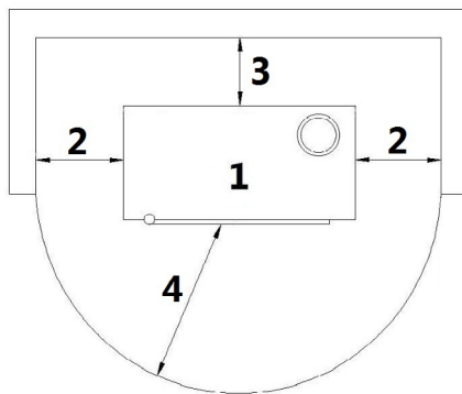
Fig. 14 - Instalação geral
