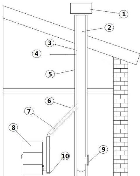
Fig. 5 - Componentes da chaminé
