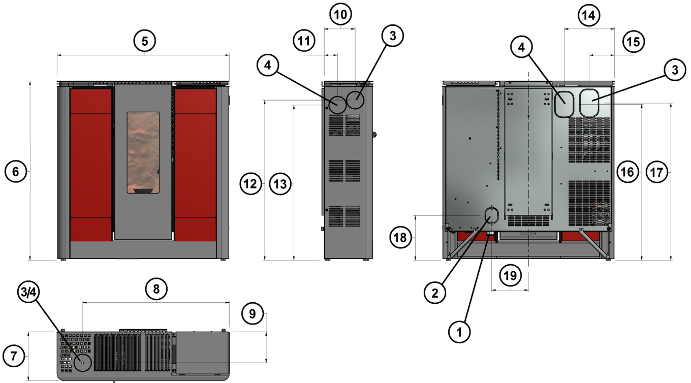
Fig. 13 - Dimensions générales: Style
