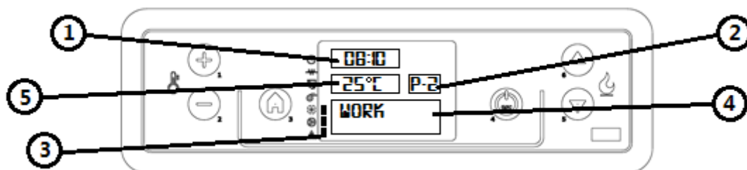
Fig. 31 - Display di controllo LCD
