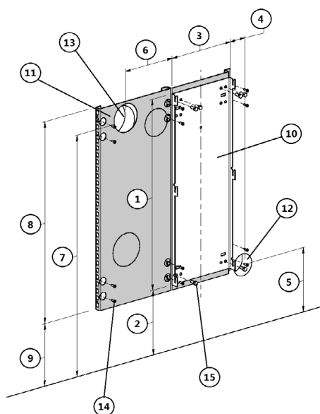
Fig. 17 - Fixation au mur inflammable
