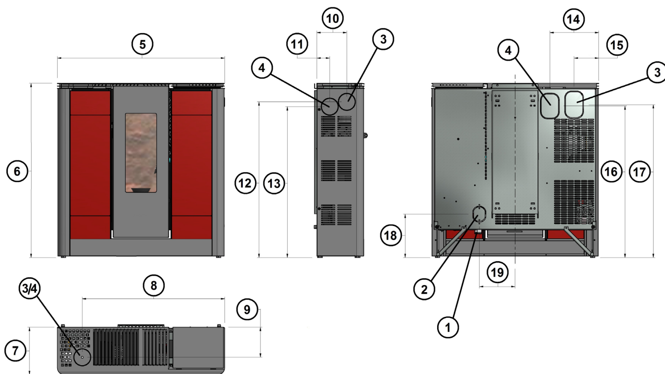
Fig. 13 - Dimensioni generali: Style
