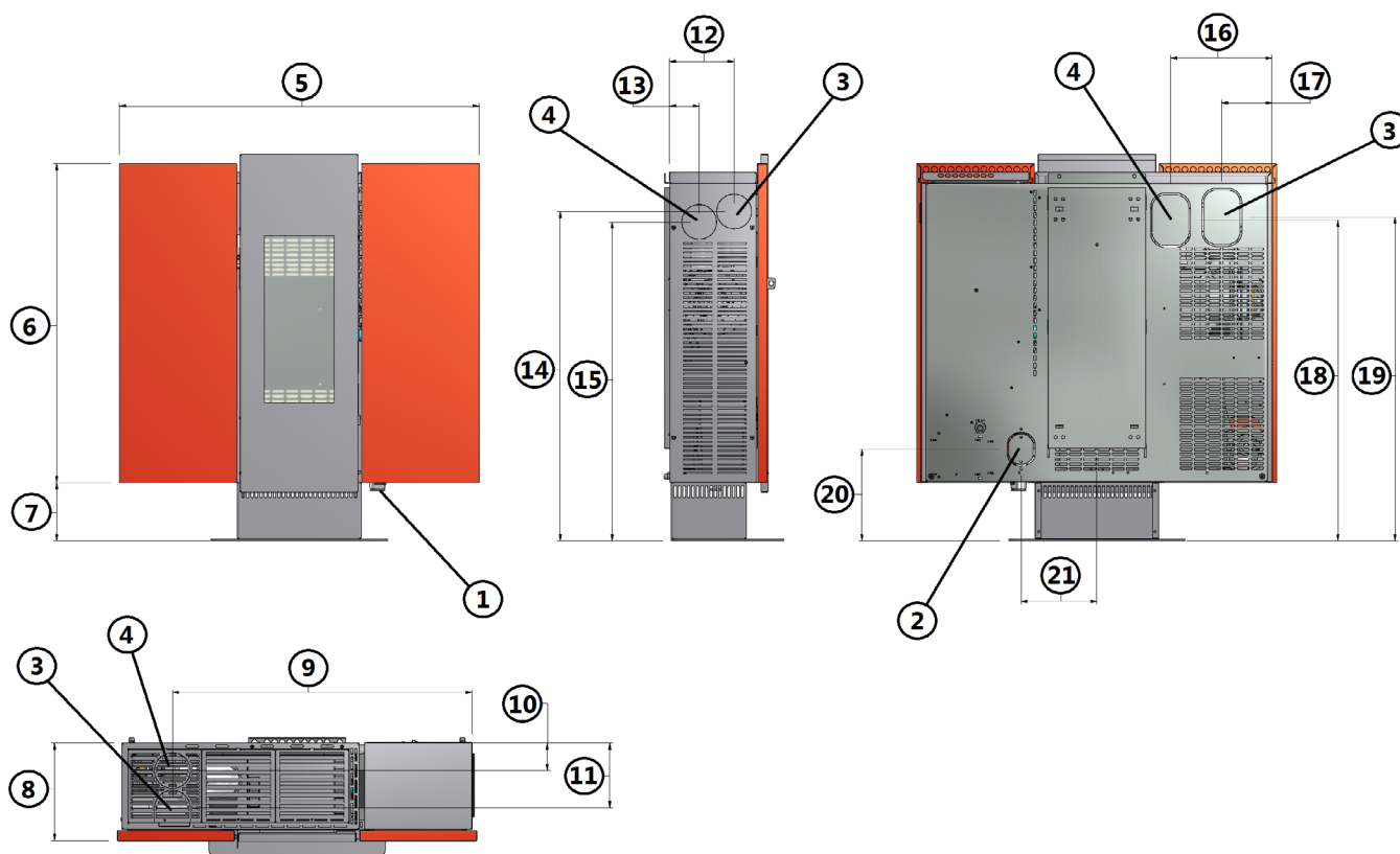
Fig. 12 - Dimensioni generali: Wall/Small
