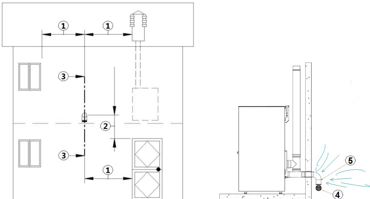
Fig. 7 - Prise d'air pour installation
