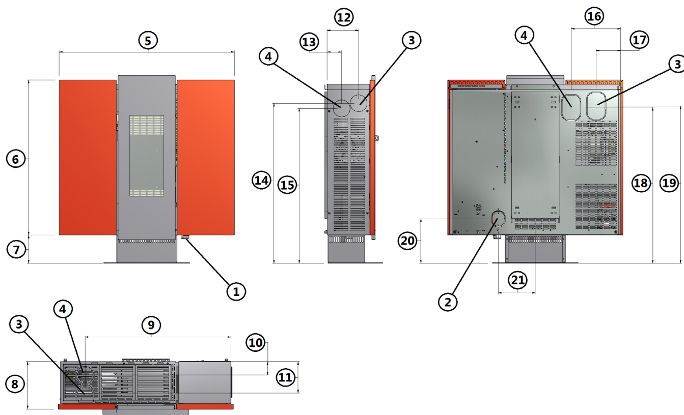
Fig. 12 - Dimensions générales: Wall/Small
