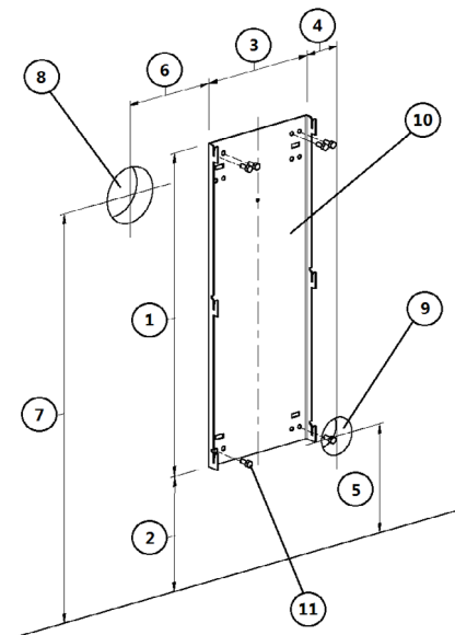
Fig. 16 - Fixation au mur non inflammable
