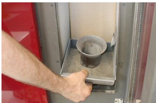
Fig. 35 - Extraction de le brasero
