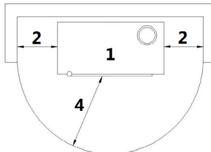
Fig. 15 - Installazione a parete
