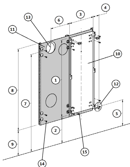
Fig. 17 - Fissaggio su parete infiammabili
