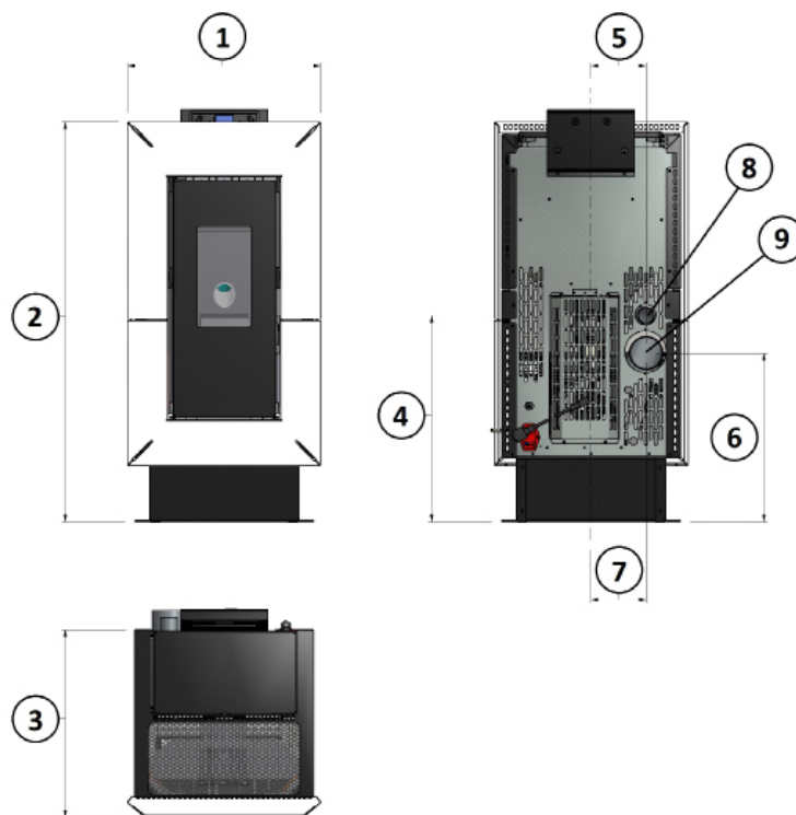
Fig. 17 - Dimensions générales: Elan
