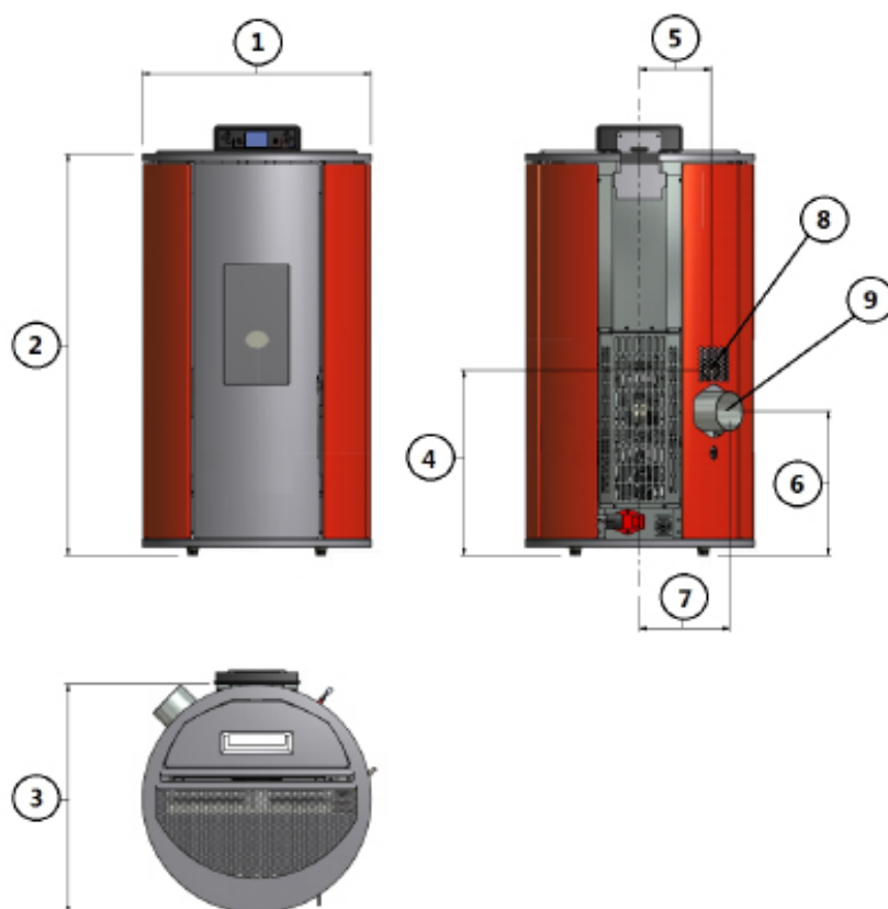
Fig. 14 - Dimensions générales: Rondò
