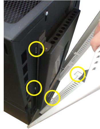
Fig. 22 - Fixation du panneau frontal
