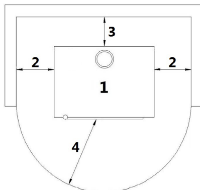
Fig. 18 - Installation générique
