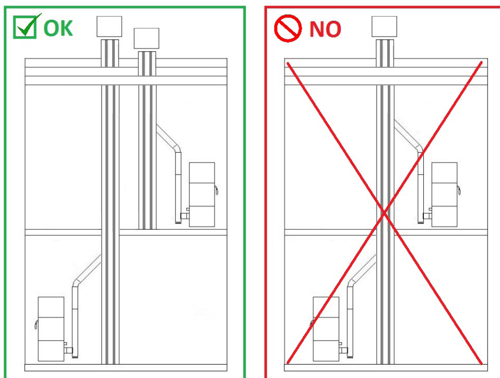
Fig. 13 - Exemples des installation correcte
