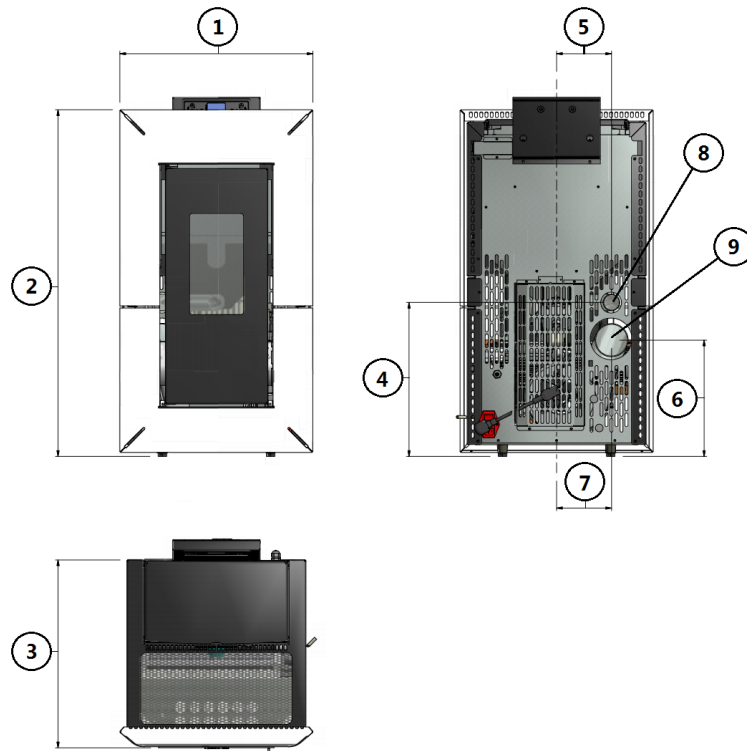
Fig. 15 - Dimensions générales: Mika
