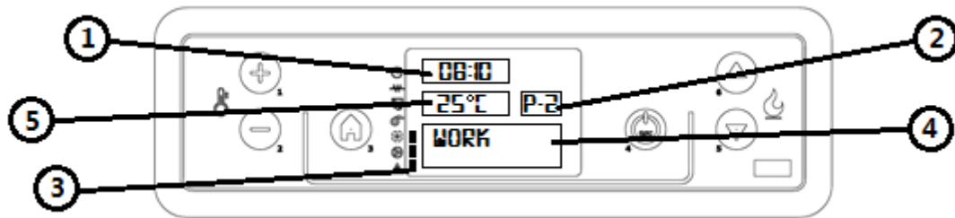
Fig. 30 - Tableau de contrôle LCD
