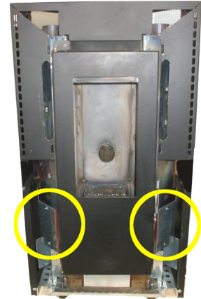
Fig. 58 - Passages des fumées
