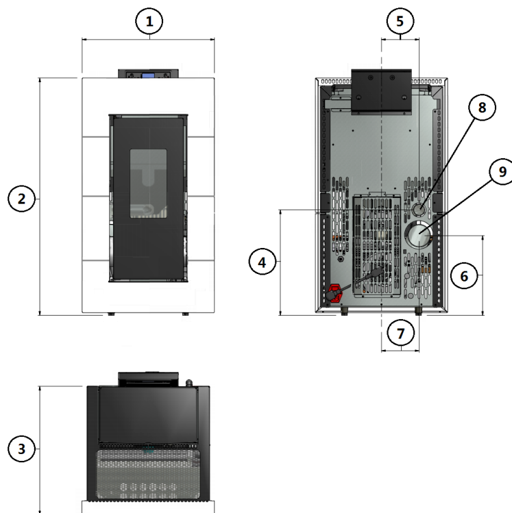
Fig. 16 - Dimensions générales: Kami
