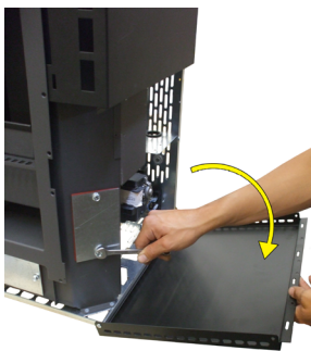
Fig. 62 - Enlever les bouchons
