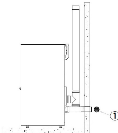
Fig. 8 - Grille de protection
