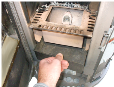
Fig. 36 - Extraction de le tiroir à cendre
