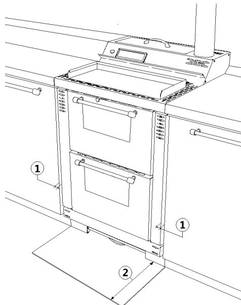
Fig. 14 - Cozinha embutida
