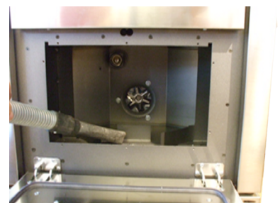
Fig. 30 - Limpeza da câmara de fumos
