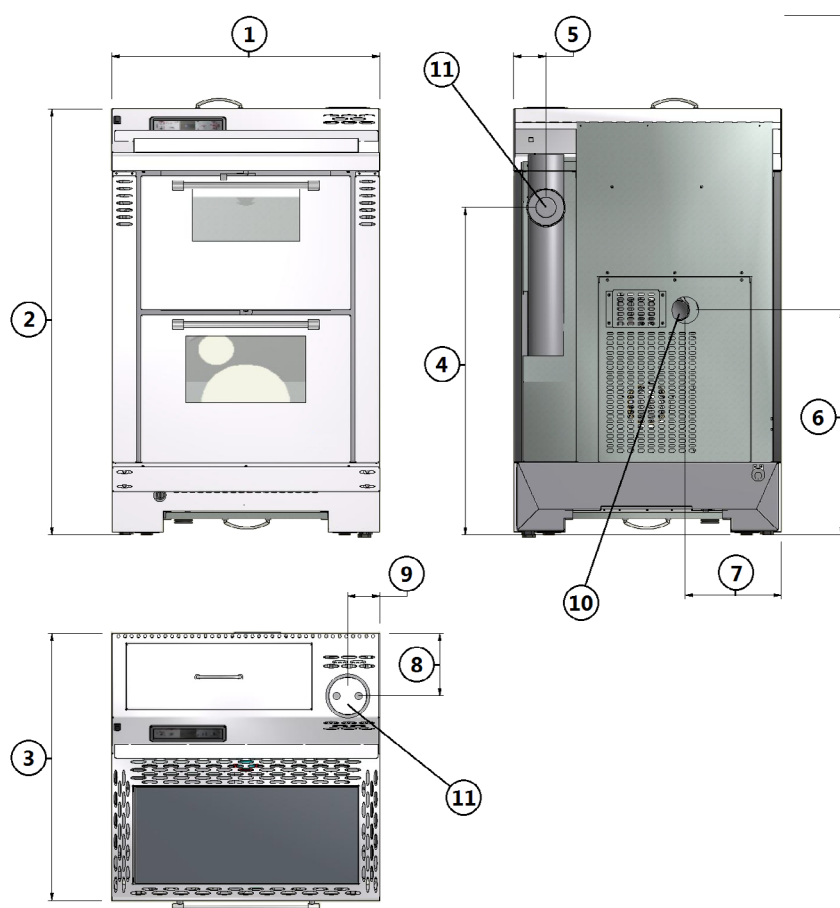
Fig. 12 - Dimensões gerais
