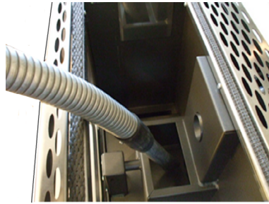
Fig. 25 - Limpeza do compartimento do braseiro
