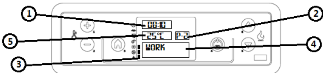
Fig. 51 - Ecrã de controlo LCD
