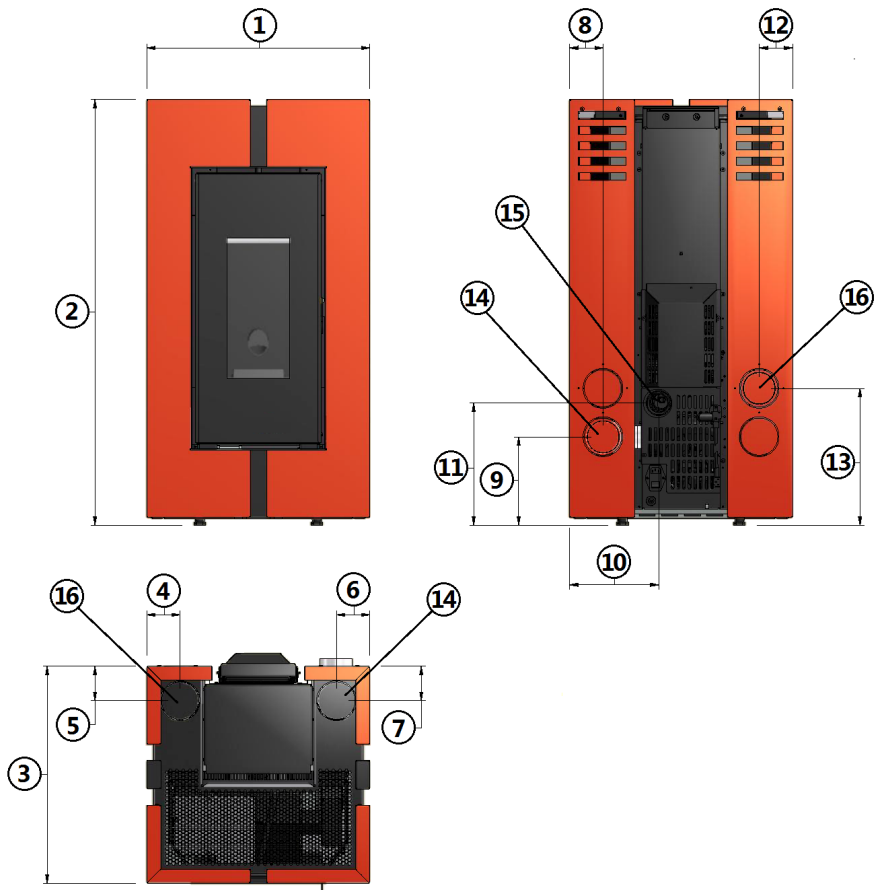
Fig. 17 - Dimensões gerais: Doge 3 Plus
