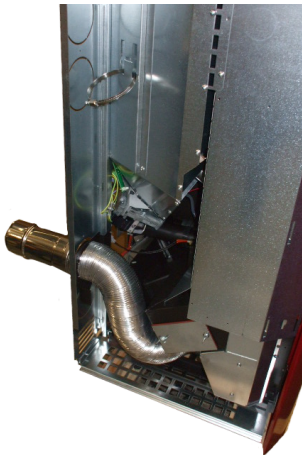
Fig. 47 - Posicionamento tubos posteriores
