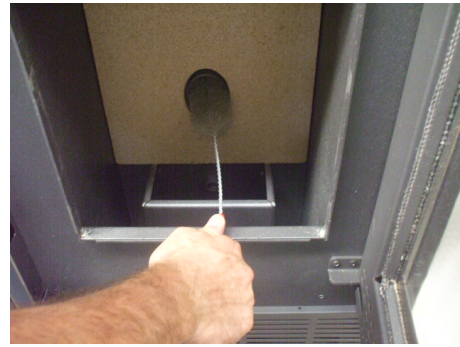
Fig. 59 - Limpeza com escova
