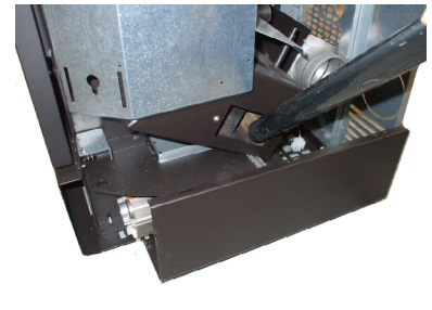
Fig. 81 - Limpeza da câmara de fumos
