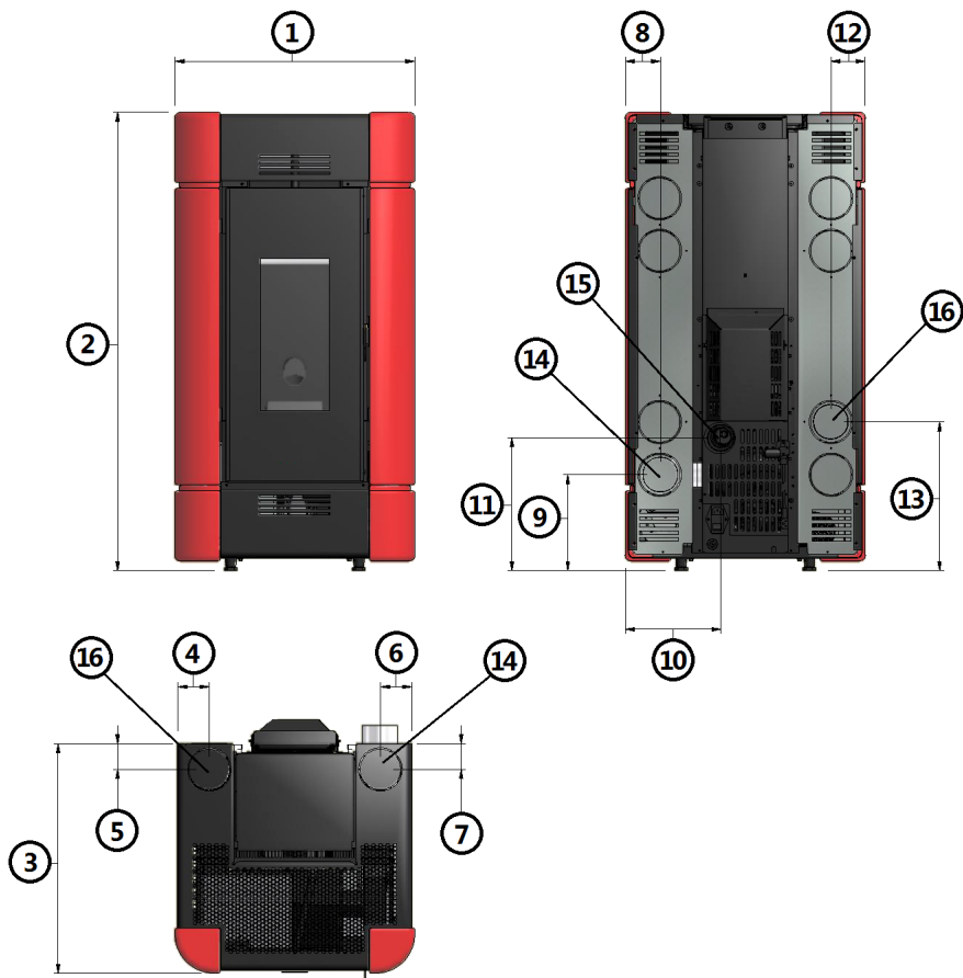
Fig. 16 - Dimensões gerais: Sire 3 Plus
