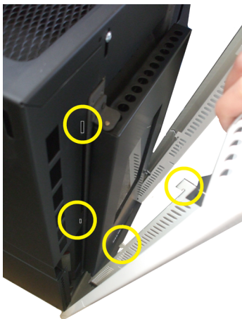
Fig. 22 - Montagem painel frontal
