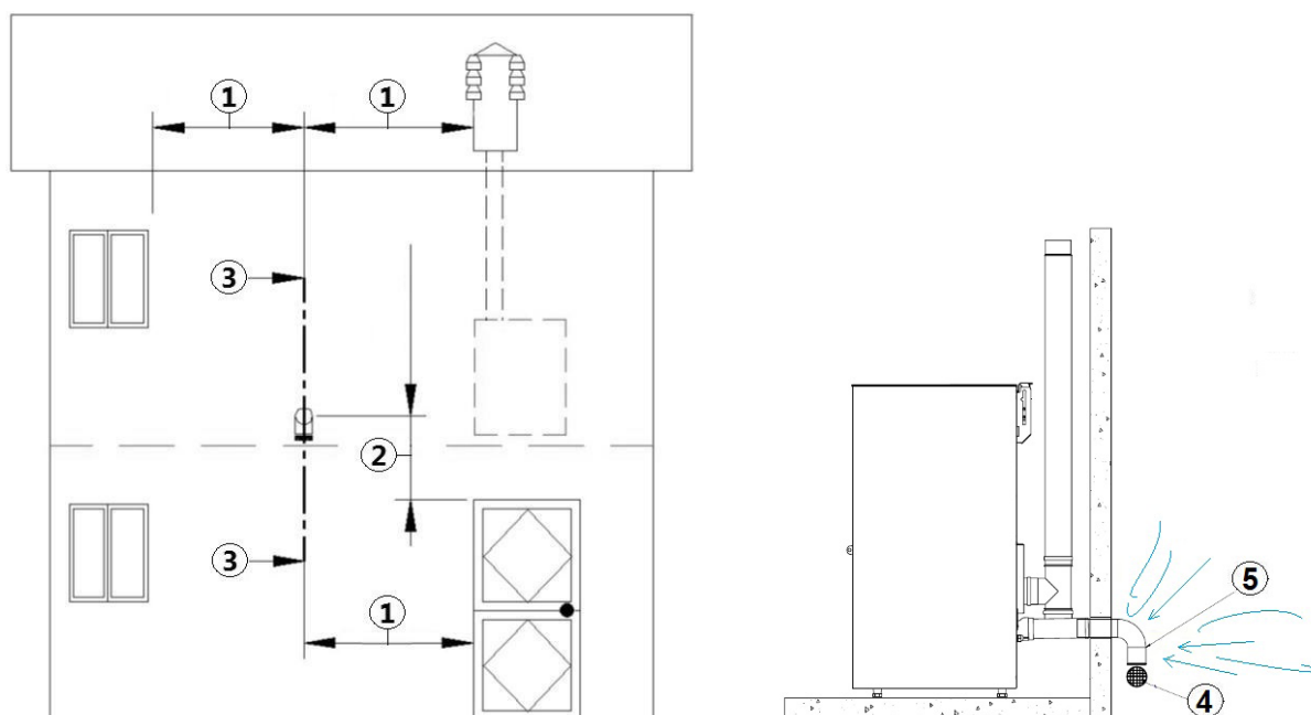
Fig. 8 - Tomada ar para instalação compartimento estanque
