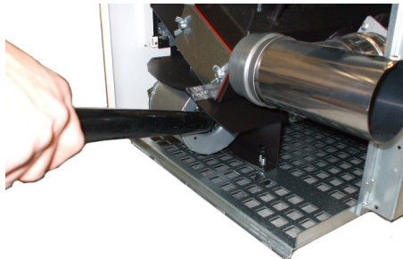
Fig. 87 - Limpeza do ventilador ambiente
