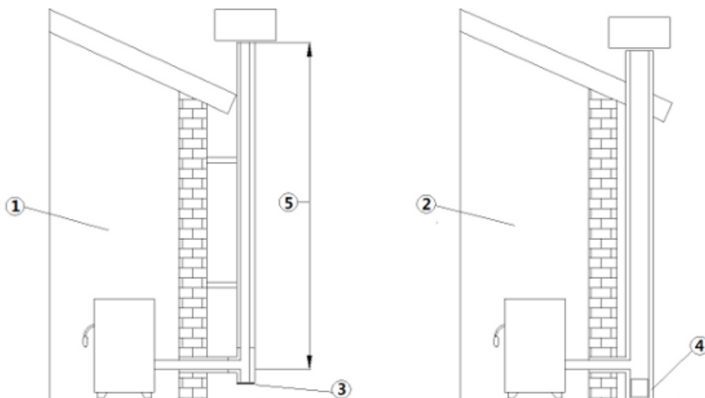
Fig. 2 - Conduitas de evacuação de fumos
