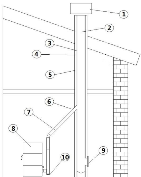
Fig. 6 - Componentes da chaminé
