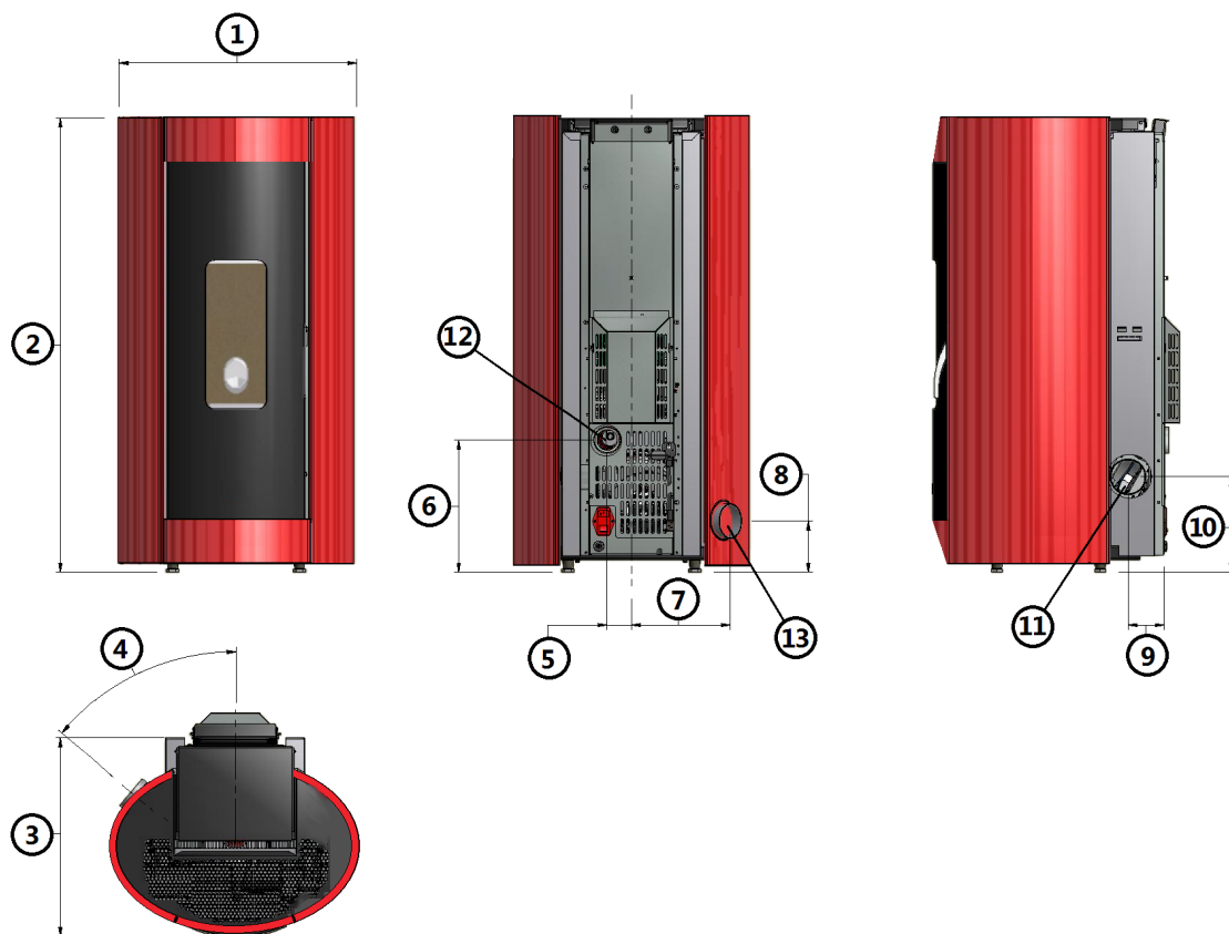
Fig. 20 - Dimensões gerais: Elise 3
