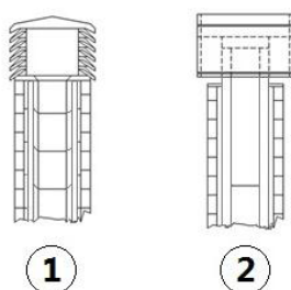
Fig. 5 - Chapéus antivento
