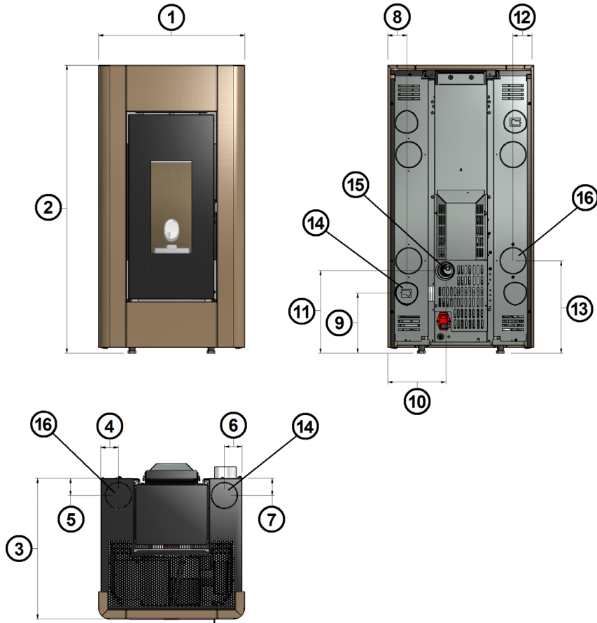
Fig. 19 - Dimensões gerais: Prince 3 / Prince 3 Plus
