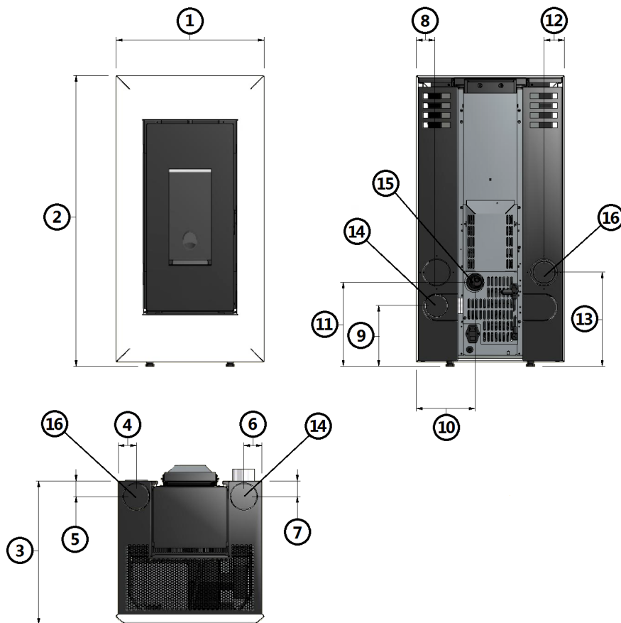
Fig. 15 - Dimensões gerais: Vega / Trend
