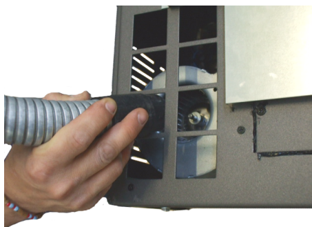
Fig. 49 - Reiniging omgevingsventilator
