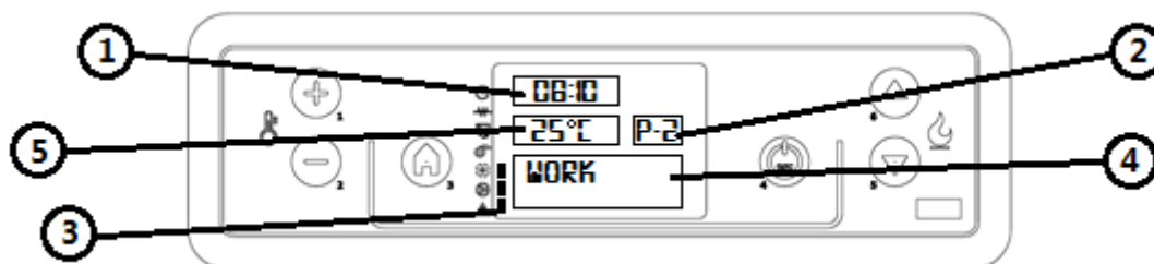
Fig. 31 - Controledisplays LCD
