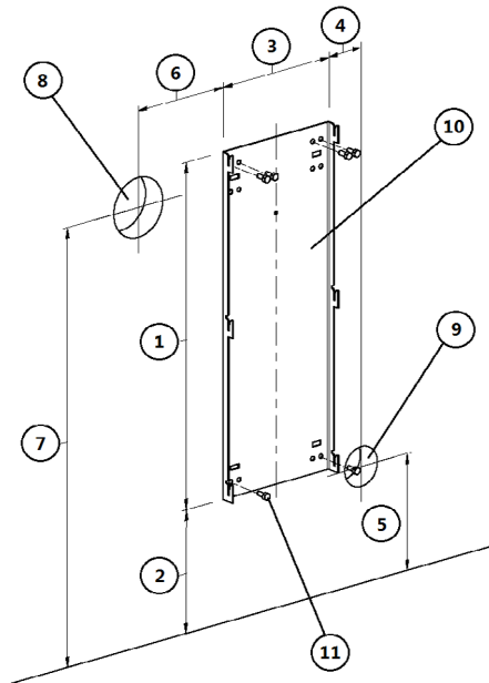
Fig. 16 - Bevestiging op niet ontvlambare muren
