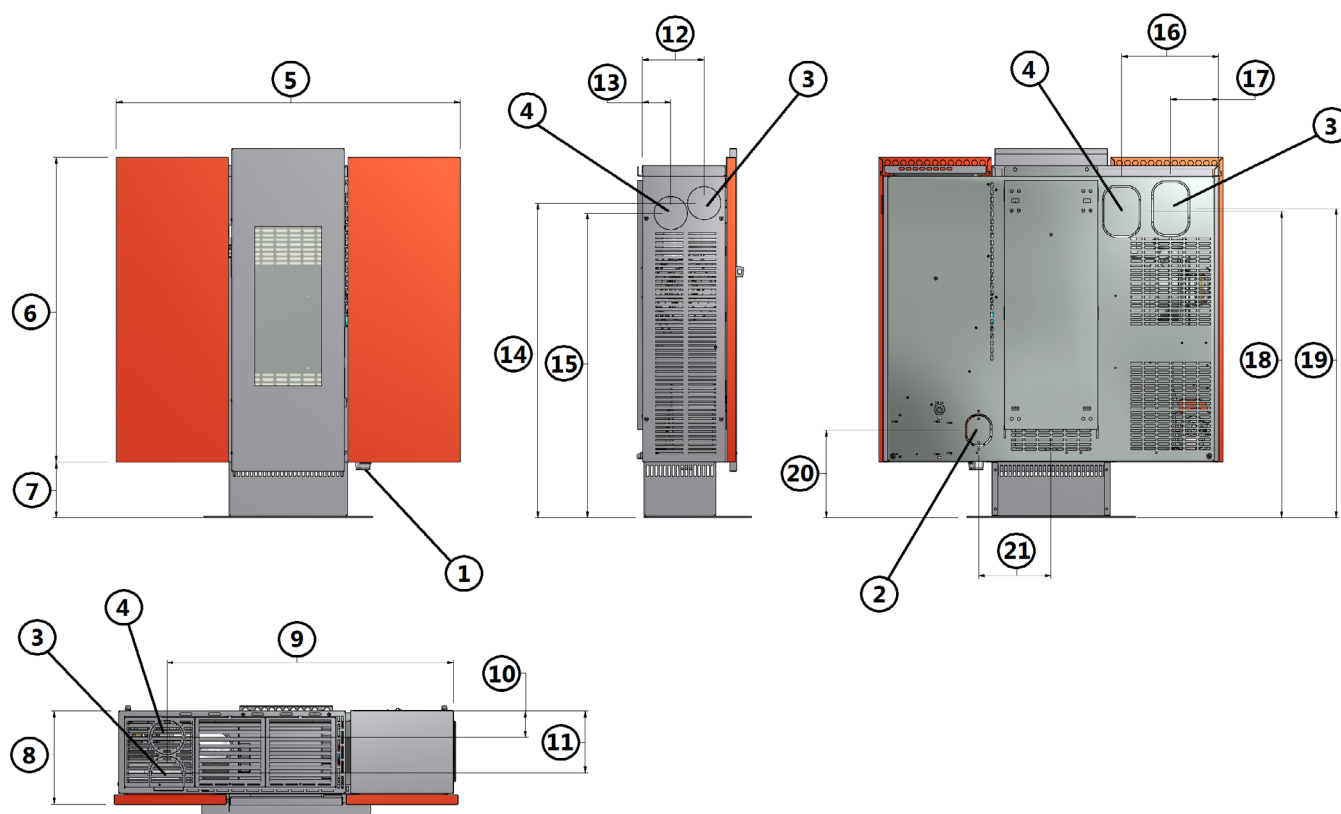
Fig. 12 - Algemene afmetingen: Wall/Small
