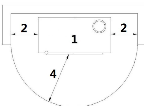
Fig. 15 - Installatie tegen de muur
