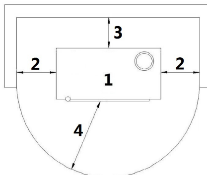
Fig. 14 - Algemene installatie
