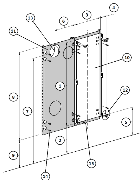
Fig. 17 - Bevestiging tegen een niet ontvlambare muur
