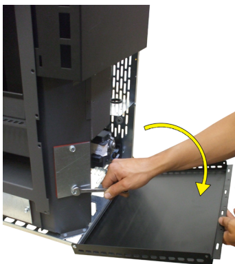
Fig. 60 - Αφαίρεση βιδών
