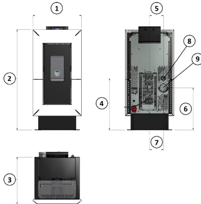
Fig. 15 - Γενικές Διαστάσεις: Elan
