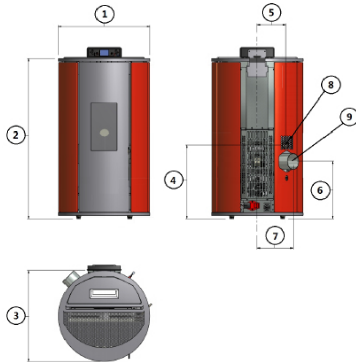
Fig. 12 - Γενικές Διαστάσεις: Rondò
