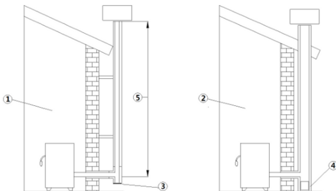
Fig. 1 - Condução de evacuação de fumos
