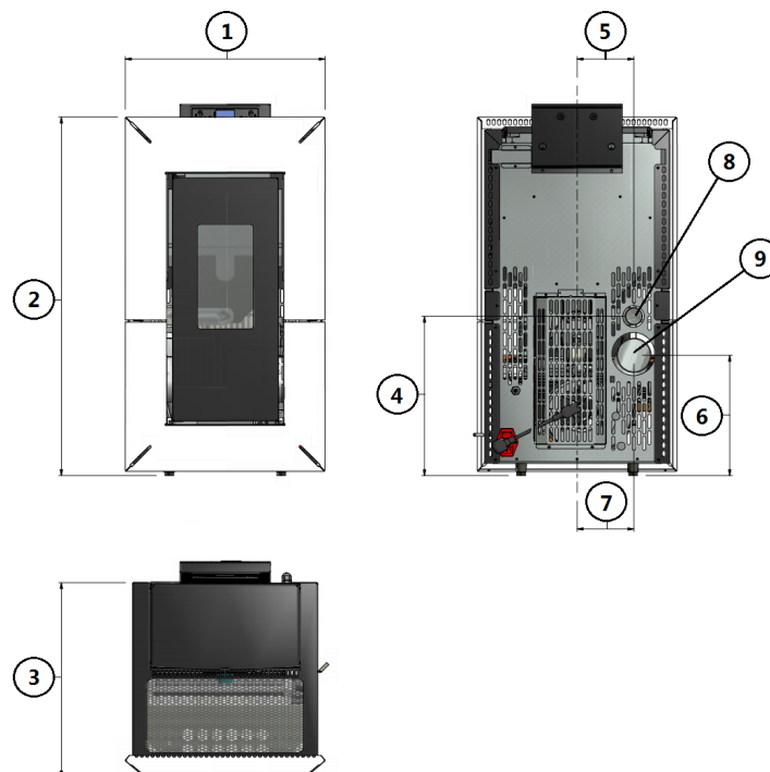
Fig. 13 - Dimensões gerais: Mika
