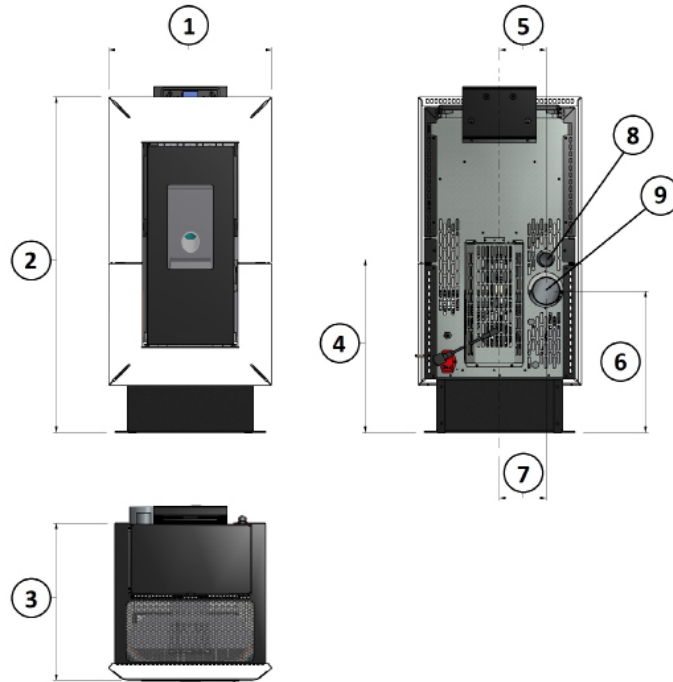
Fig. 15 - Dimensões gerais: Elan
