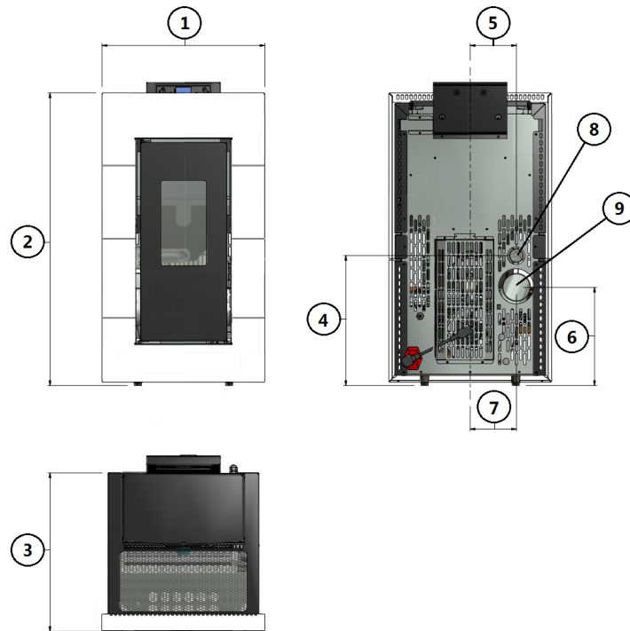
Fig. 14 - Dimensões gerais: Kami
