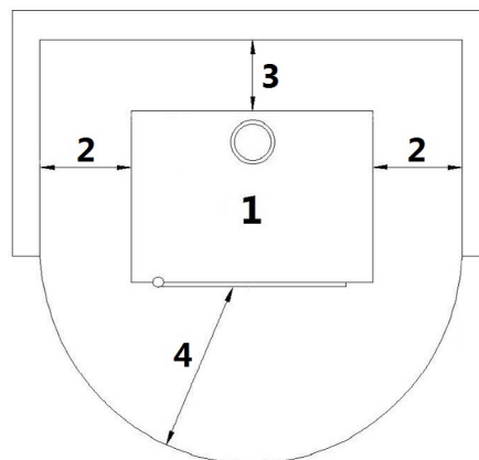
Fig. 16 - Instalação geral
