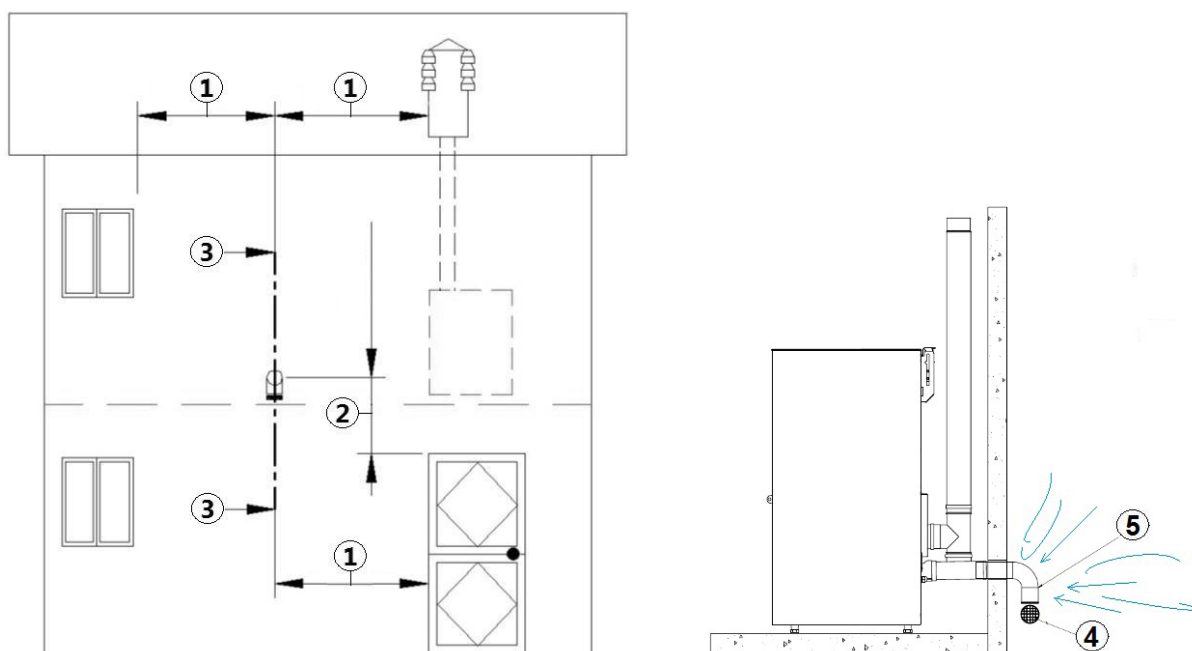
Fig. 8 - Presa d'aria per installazione a camera stagna
