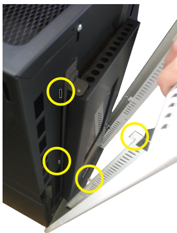
Fig. 22 - Montaggio cornice
