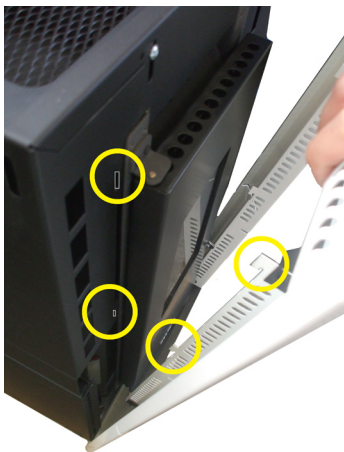
Fig. 36 - Montaggio cornice
