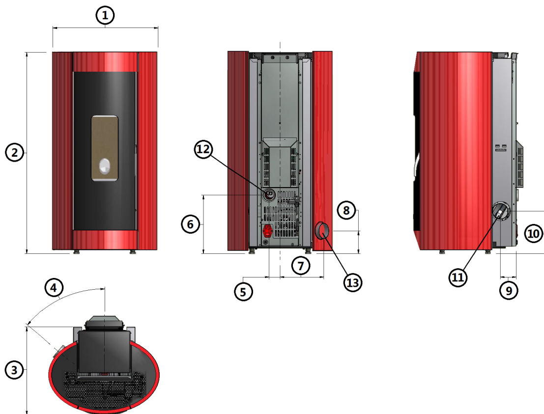
Fig. 20 - Dimensioni generali: Elise 3 Plus
