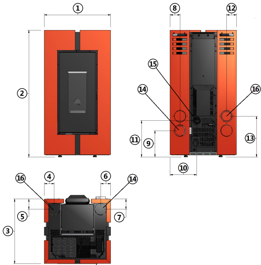
Fig. 17 - Dimensioni generali: Doge 3 Plus
