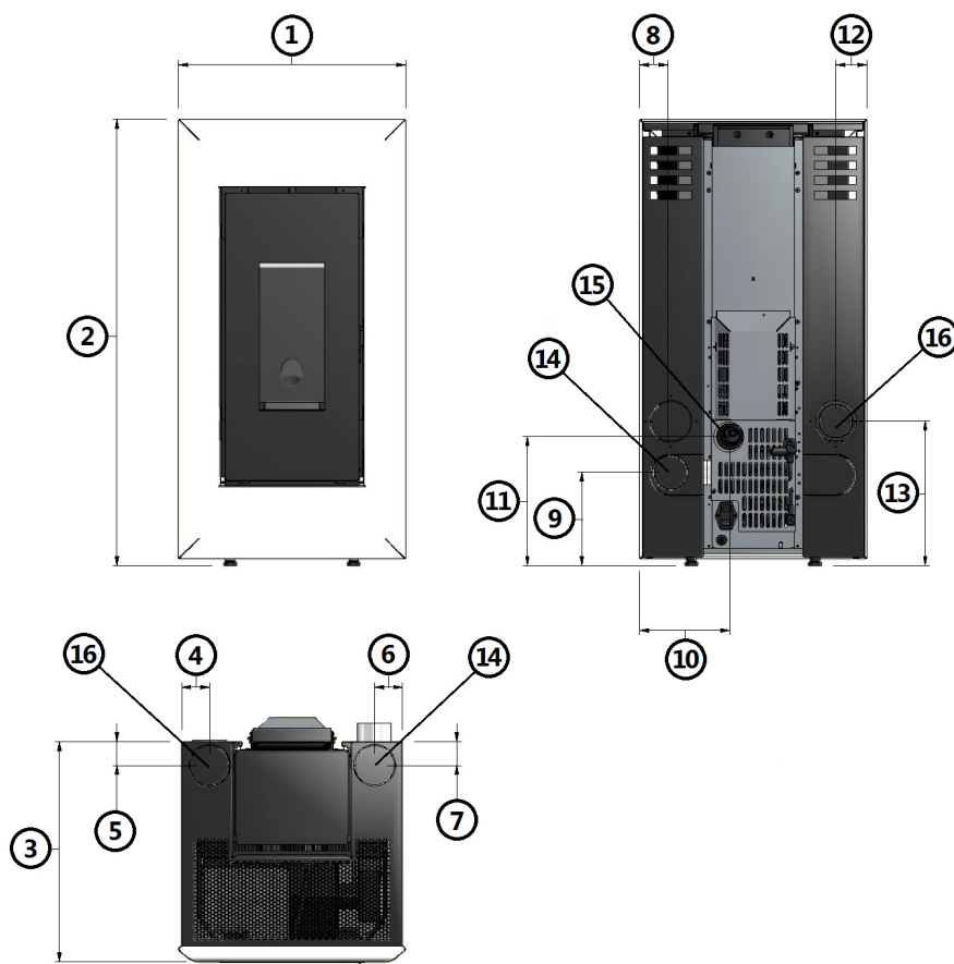
Fig. 15 - Dimensioni generali: Vega / Trend
