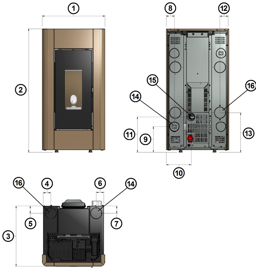
Fig. 19 - Dimensioni generali: Prince 3 / Prince 3 Plus
