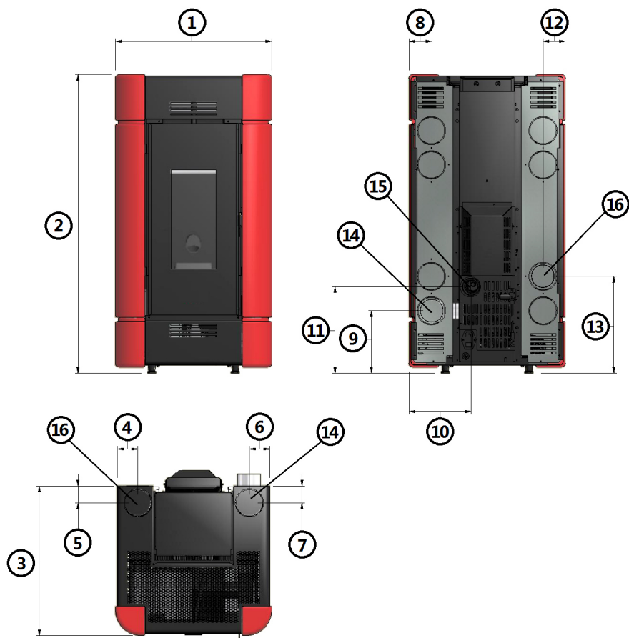
Fig. 16 - Dimensioni generali: Sire 3 Plus
