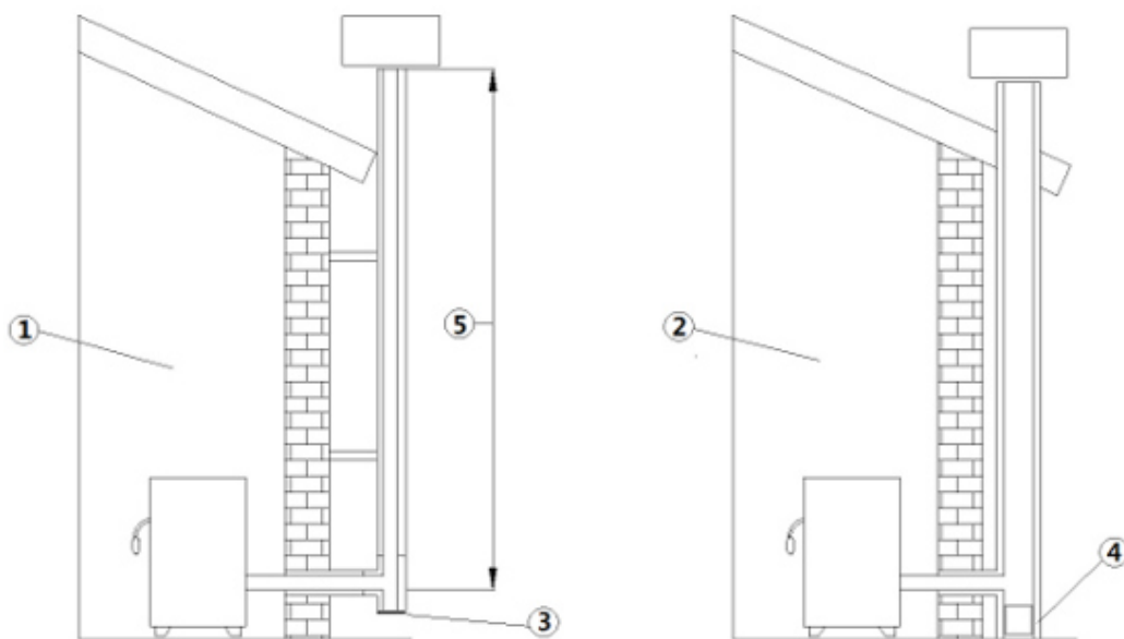
Fig. 2 - Canne fumarie
