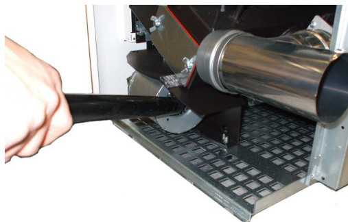
Fig. 87 - Pulizia ventilatore ambiente
