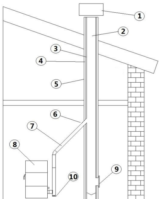
Fig. 6 - Componenti camino
