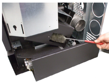
Fig. 80 - Pulizia con scovolino 2
