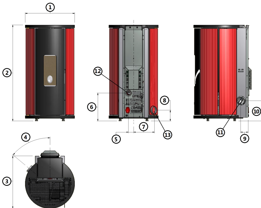
Fig. 18 - Dimensioni generali: Sfera 3 / Sfera 3 Plus / Globe
