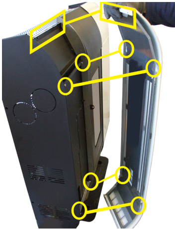
Fig. 20 - Inserción de los paneles
