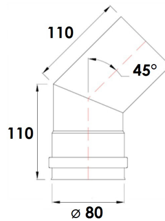
Fig. 13 - Curva a 45°
