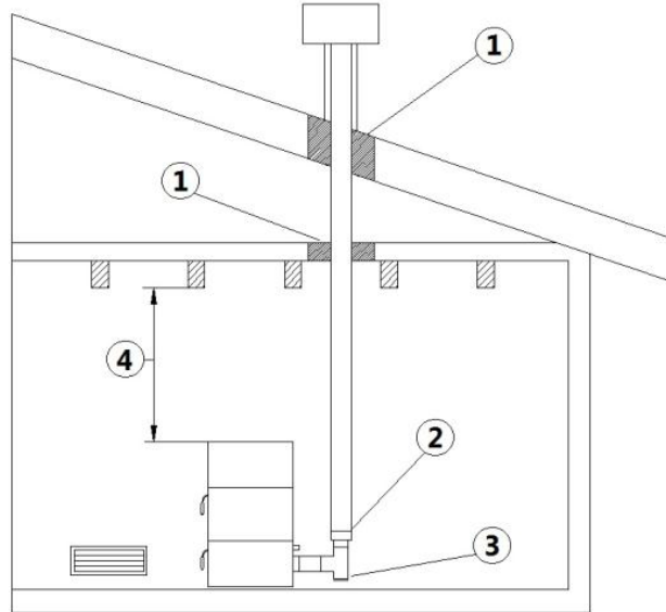
Fig. 8 - Ejemplo 1
