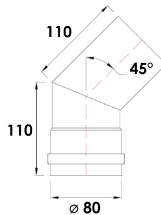
Fig. 13 - Curva 45°
