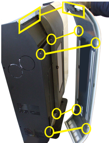
Fig. 20 - Inserção painéis
