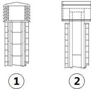
Fig. 4 - Extremos de chimenea antiviento
