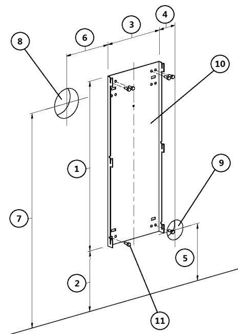
Fig. 18 - Fixação em parede não inflamável
