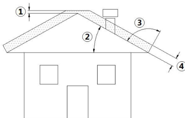
Fig. 2 - Teto inclinado
