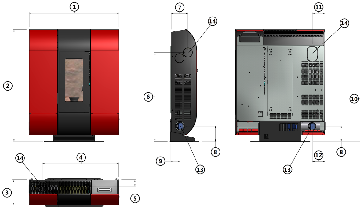
Fig. 11 - Dimensões gerais
