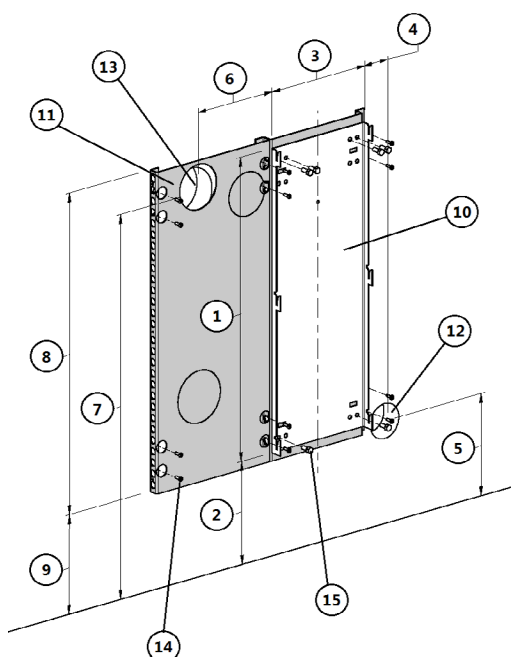
Fig. 19 - Fijación en pared inflamable
