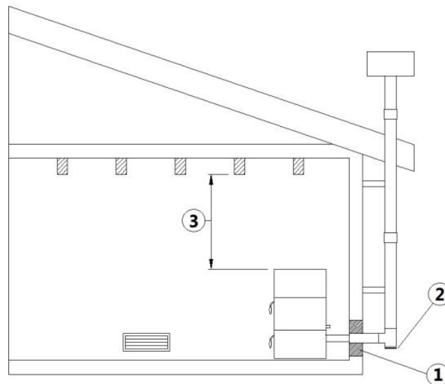
Fig. 10 - Exemplo 3
