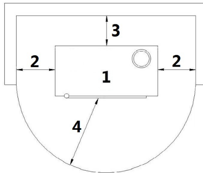
Fig. 14 - Instalación genérica con pedestal
