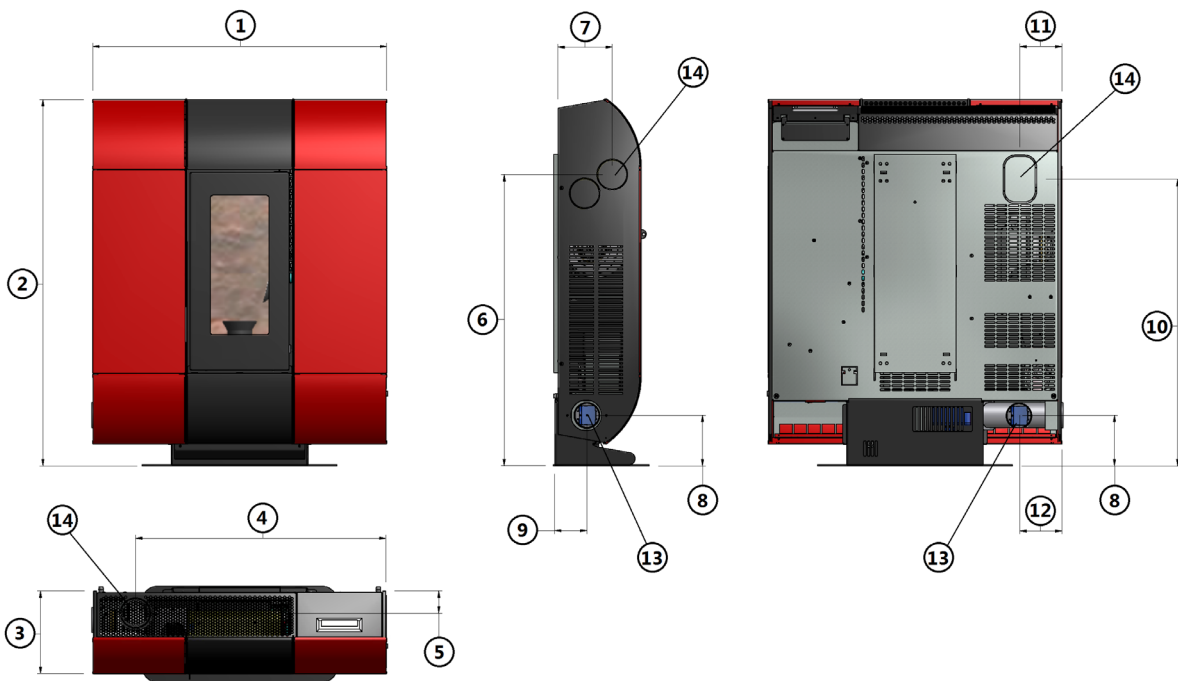
Fig. 11 - Dimensiones generales
