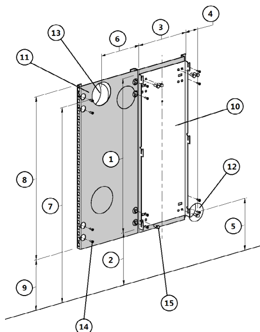
Fig. 19 - Fixação em parede não inflamável
