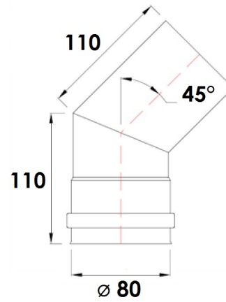
Fig. 16 - Curva 45°
