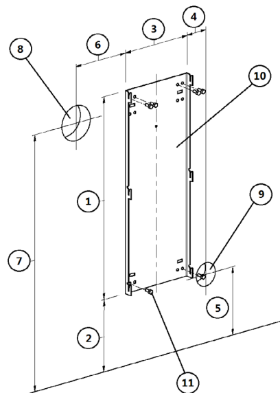
Fig. 18 - Fijación en pared no inflamable
