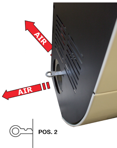
Fig. 29 - Posición de la palanca para desviar el aire: pos. 2
