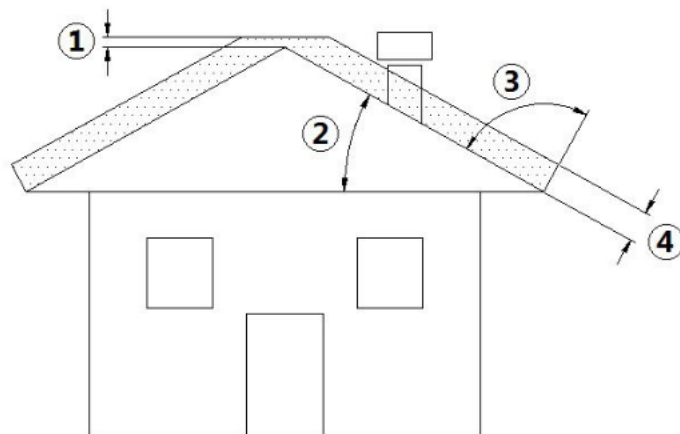
Fig. 2 - Techo inclinado
