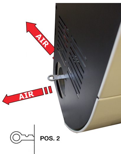
Fig. 29 - Posição da alavanca para o desvio do ar: pos.2
