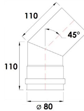
Fig. 16 - Curva a 45°
