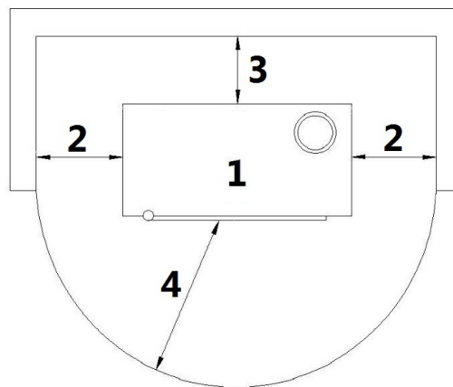
Fig. 14 - Instalação geral com base
