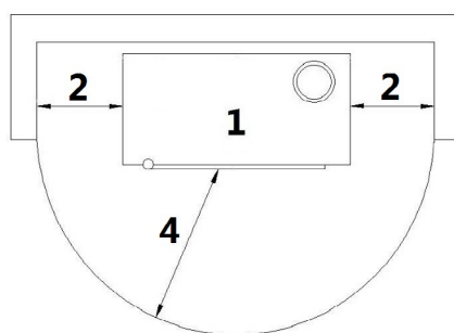
Fig. 17 - Installatie tegen de muur
