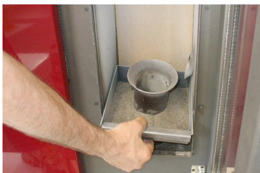
Fig. 37 - Verwijdering vuurpot
