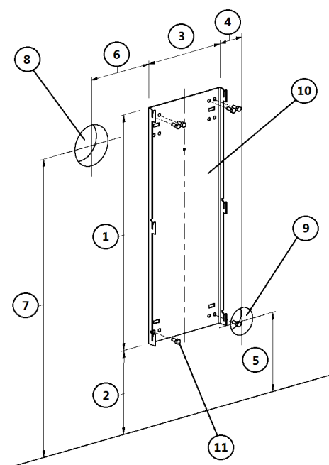
Fig. 18 - Bevestiging op niet ontvlambare muren
