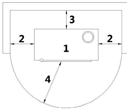
Fig. 14 - Algemene installatie met voetstuk
