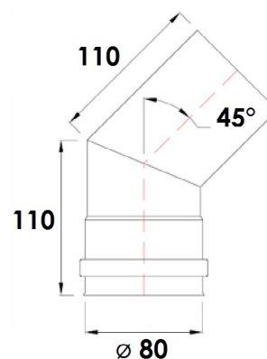
Fig. 13 - Bochten 45°
