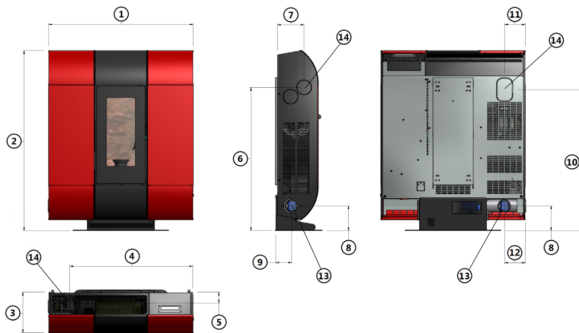
Fig. 11 - Algemene afmetingen
