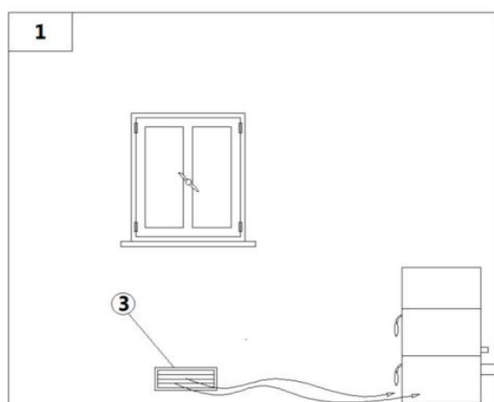
Fig. 6 - Directe luchthoevoer
