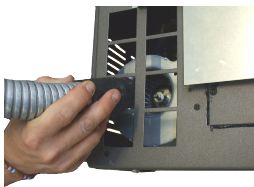
Fig. 50 - Room fan cleaning
