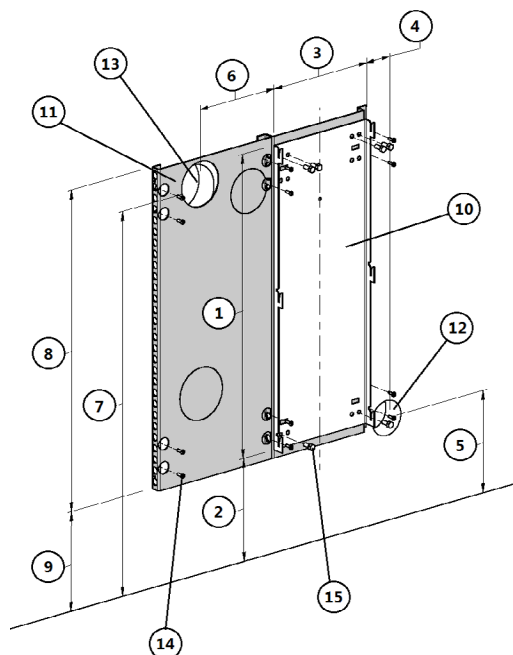
Fig. 19 - Bevestiging tegen een niet ontvlambare muur
