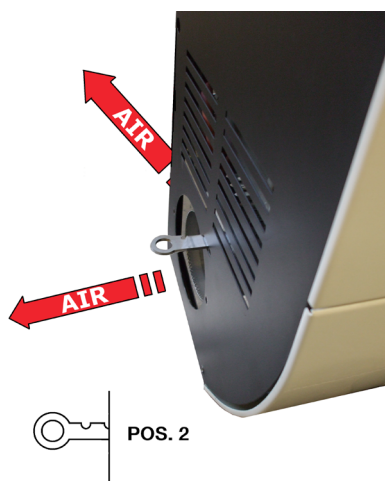
Fig. 29 - Positie van de hendel voor omleiding van de lucht: pos.2
