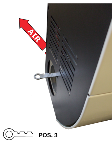
Fig. 27 - Positie van de hendel voor omleiding van de lucht: pos.3
