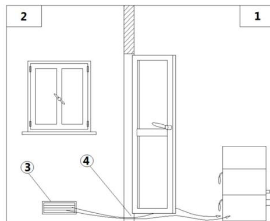
Fig. 7 - Indirecte luchthoevoer
