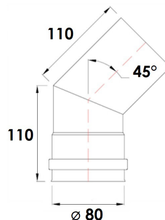
Fig. 16 - Bochten 45°
