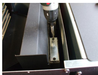
Fig. 44 - Verwijdering doppen
