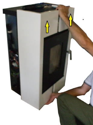
Fig. 22 - Panelen wegnemen: fase 1
