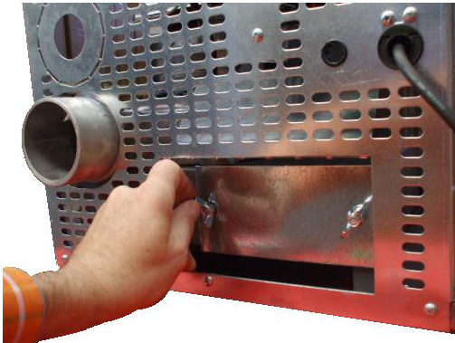
Fig. 37 - Rookgassenkamer
