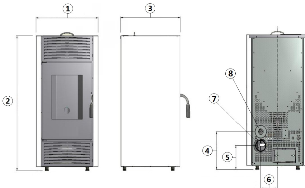
Fig. 11 - Algemene afmetingen
