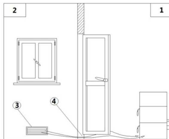
Fig. 7 - Indirecte luchthoevoer
