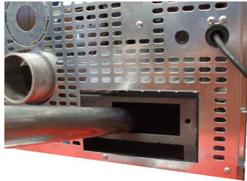
Fig. 38 - Reiniging rookgassenkamer
