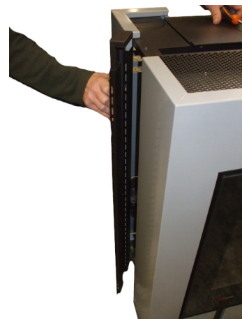
Fig. 68 - Retrait panneau central
