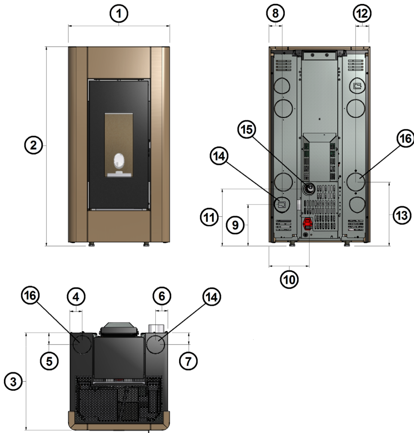
Fig. 22 - Dimensions générales: Prince 3 / Prince 3 Plus
