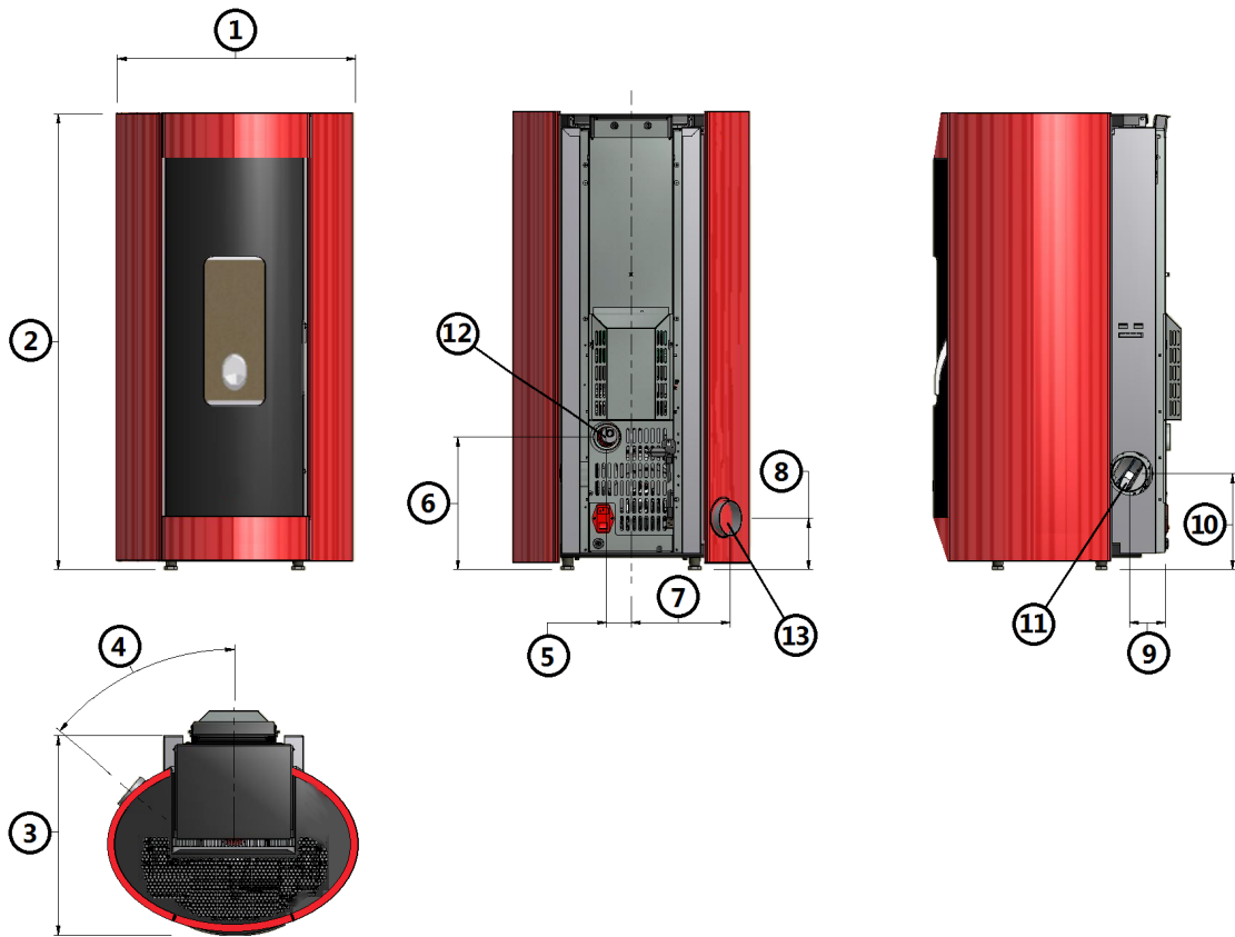
Fig. 23 - Dimensions générales: Elise 3 Plus
