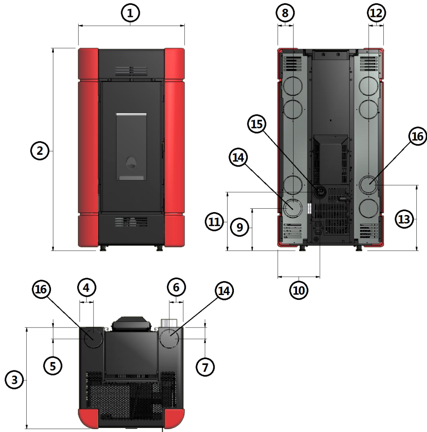
Fig. 19 - Dimensions générales: Sire 3 Plus
