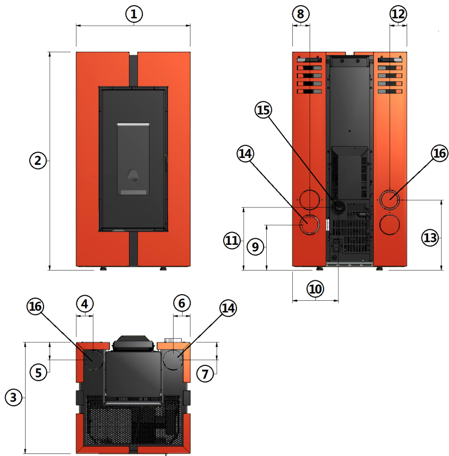
Fig. 20 - Dimensions générales: Doge 3 Plus
