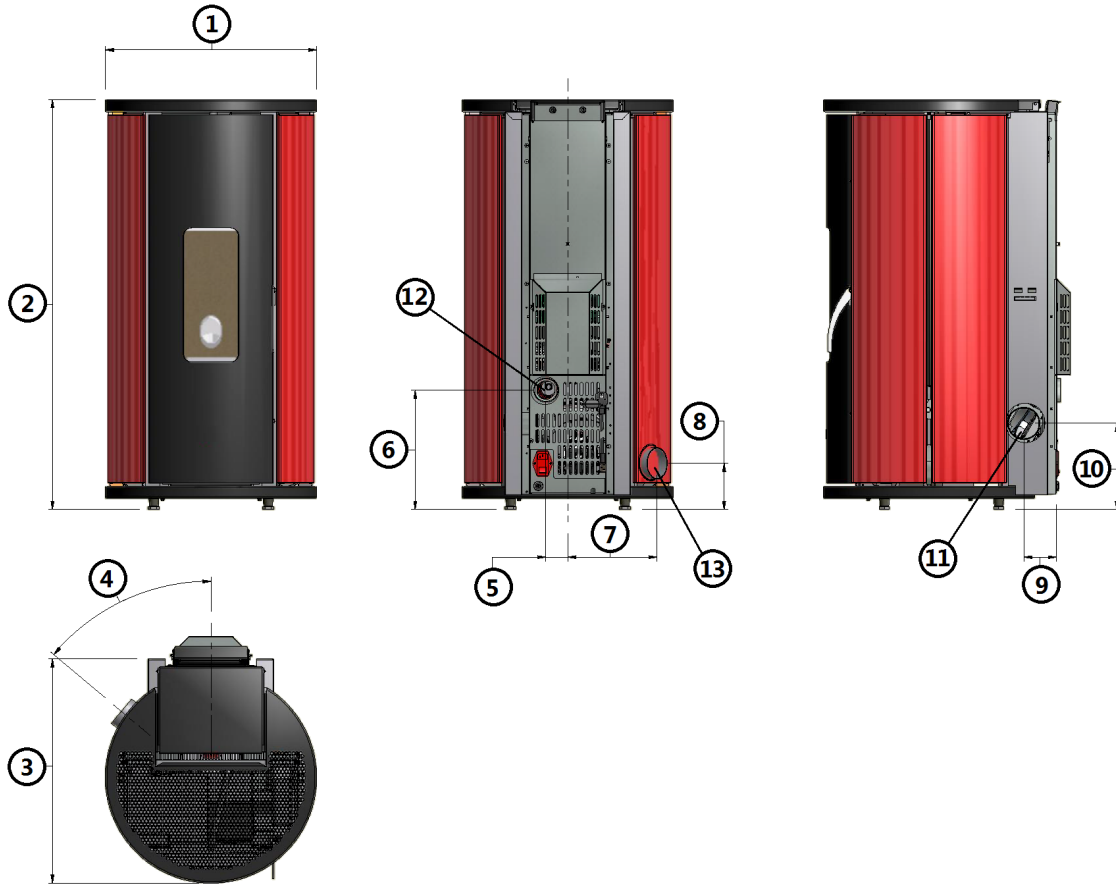
Fig. 21 - Dimensions générales: Sfera 3 / Sfera 3 Plus / Globe
