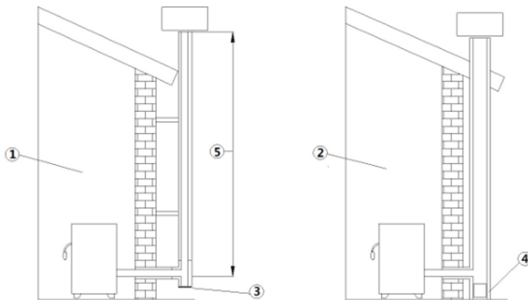
Fig. 1 - Canne fumarie
