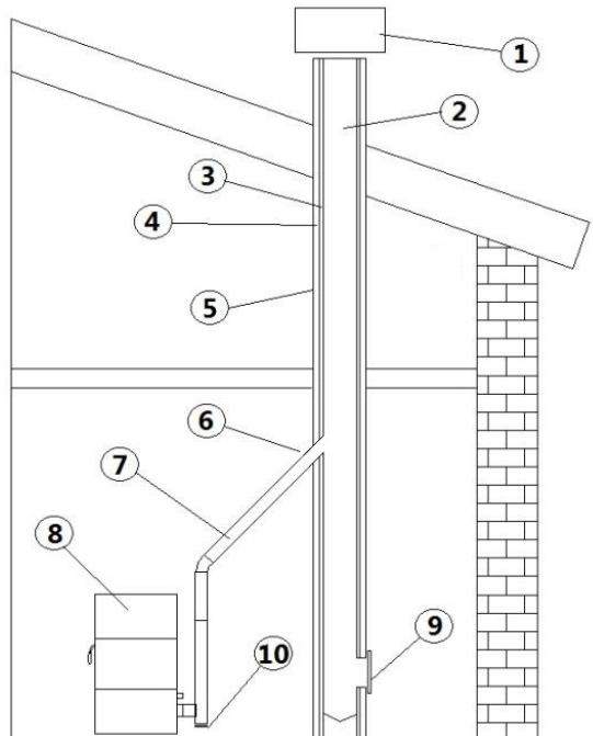
Fig. 5 - Componenti camino
