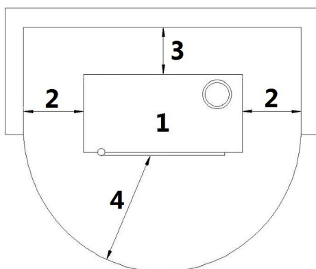
Fig. 15 - Installazione generica con piedistallo
