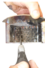
Fig. 29 - Καθαρισμός δοχείου καύσης
