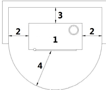
Fig. 15 - Γενική Εγκατάσταση με βάση στήριξης
