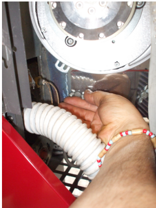
Fig. 34 - Θάλαμος καυσαερίων
