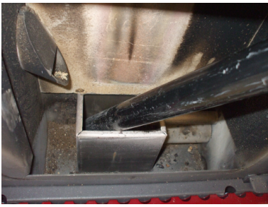
Fig. 30 - Καθαρισμός εσωτερικού μέρους δοχείου καύσεως
