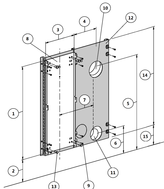
Fig. 20 - Στήριξη σε εύφλεκτο τοίχο
