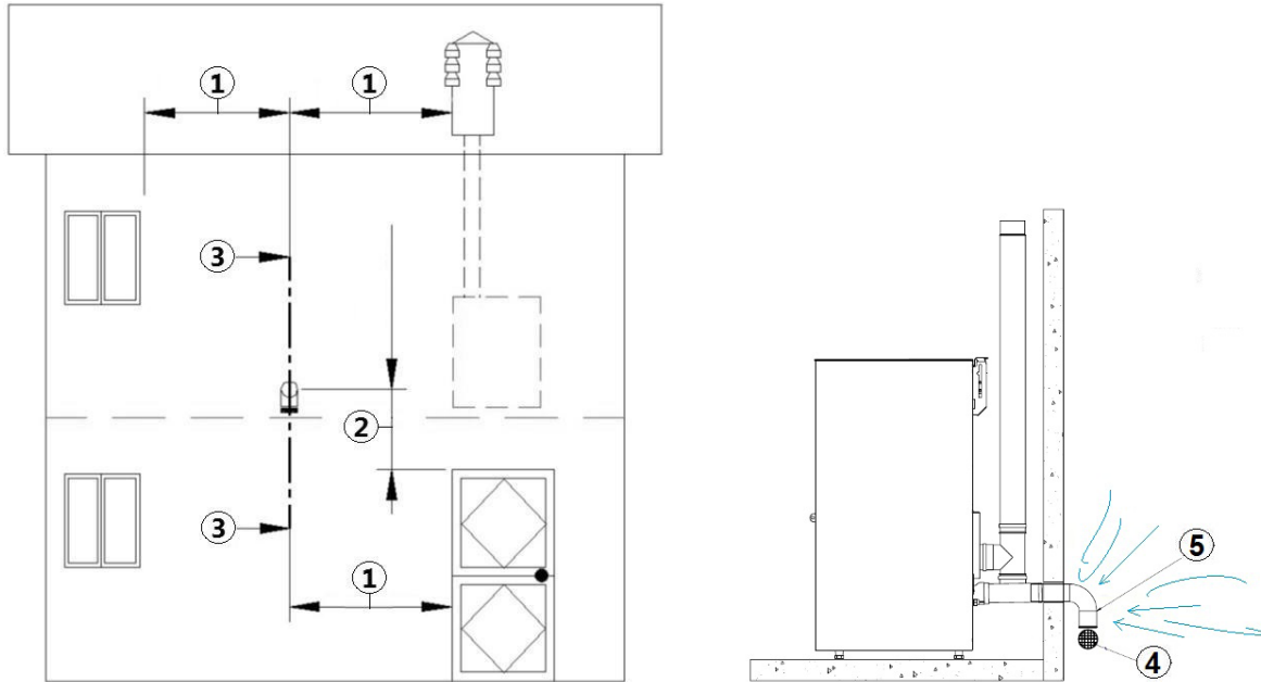
Fig. 7 - Είσοδος αέρα για εγκατάσταση σφραγισμένου θαλάμου
