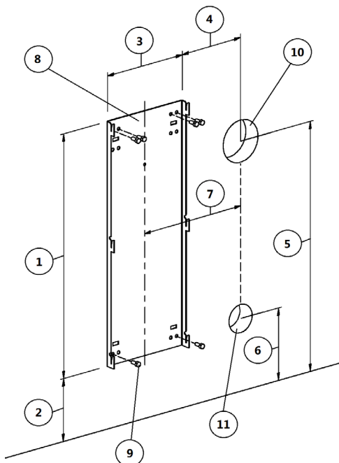
Fig. 19 - Στήριξη σε μη εύφλεκτο τοίχο
