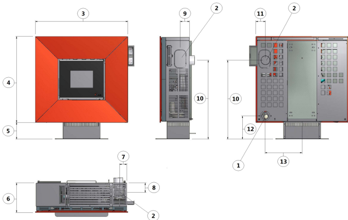
Fig. 14 - Γενικές διαστάσεις
