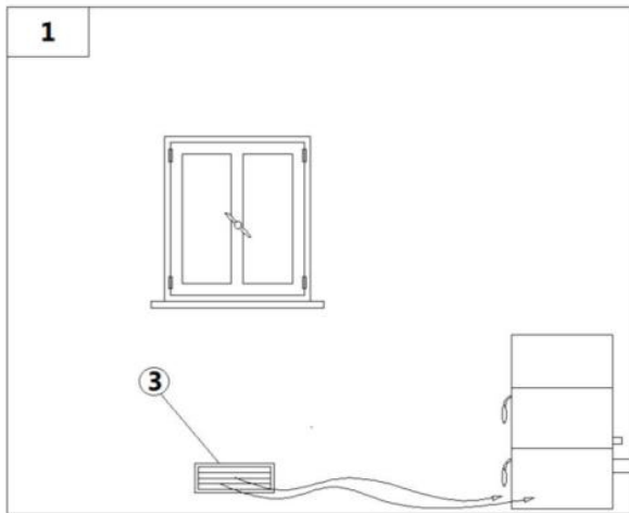
Fig. 6 - Direkte Luftzufuhr
