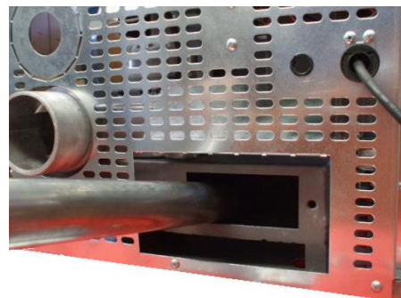
Fig. 38 - Reinigung Rauchgaskammer
