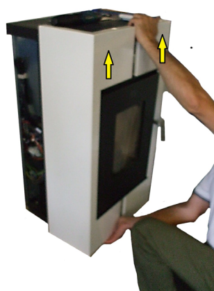
Fig. 22 - Herausziehen der Seitenwände: Phase 1
