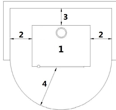
Fig. 12 - Allgemeine Installation
