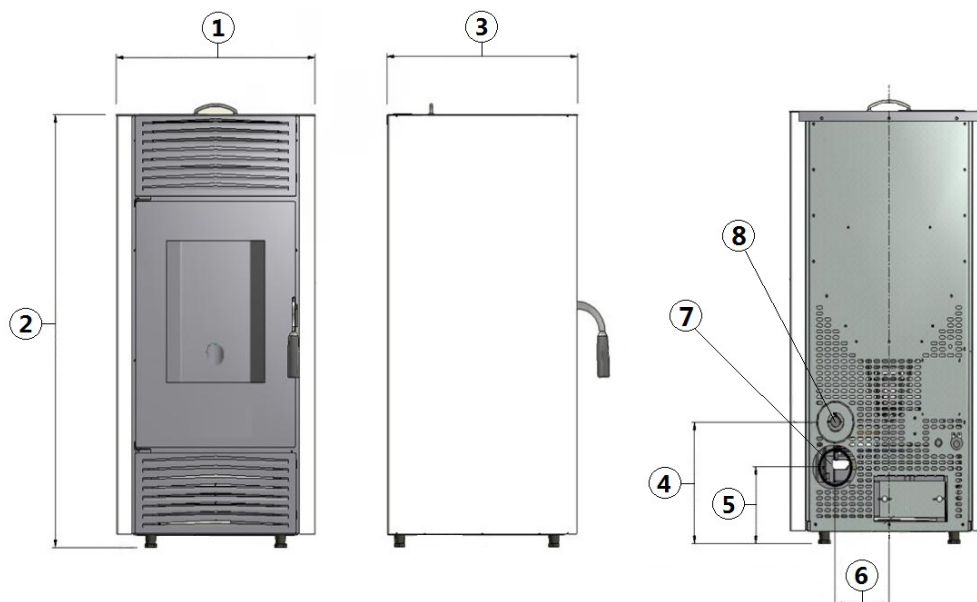
Fig. 11 - Allgemeine Abmessungen
