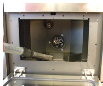
Fig. 29 - Pulizia camera fumi
