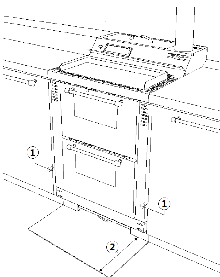
Fig. 14 - Cuisine encastrée
