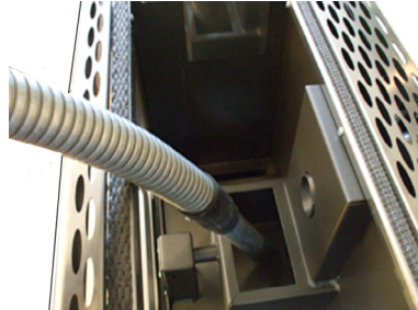
Fig. 24 - Pulizia vano braciere
