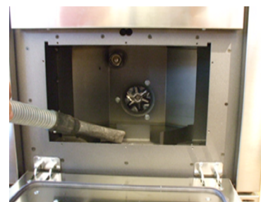
Fig. 29 - Nettoyage de la chambre des fumées
