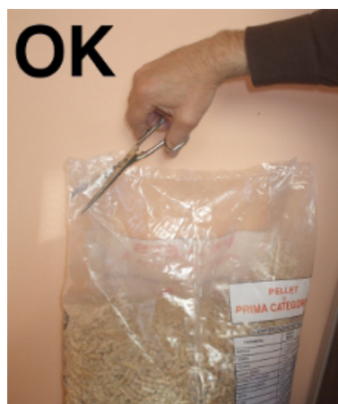
Fig. 18 - Ouverture correcte du sac des granulés
