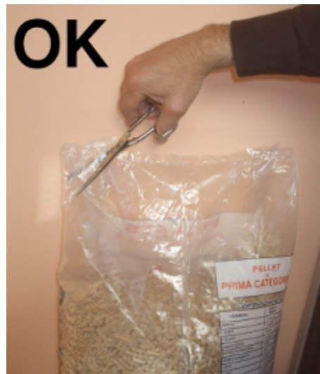
Fig. 18 - Apertura corretta del sacco di pellet
