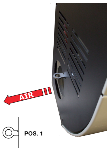
Fig. 32 - Hebelposition für die Luftableitung: Pos.1
