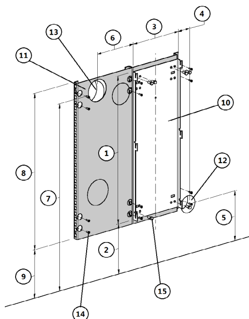
Fig. 19 - Befestigung an einer brennbaren Wand
