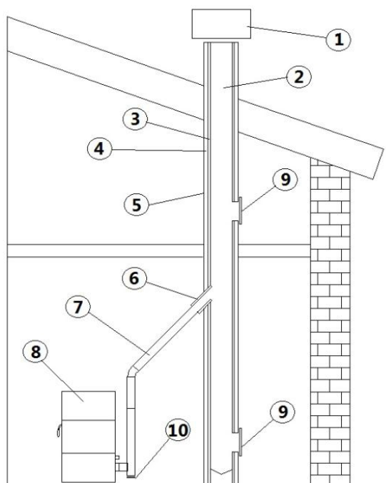
Fig. 5 - Bauteile Kamin
