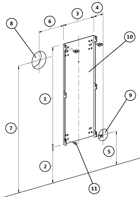
Fig. 18 - Befestigung an einer nicht brennbaren Wand
