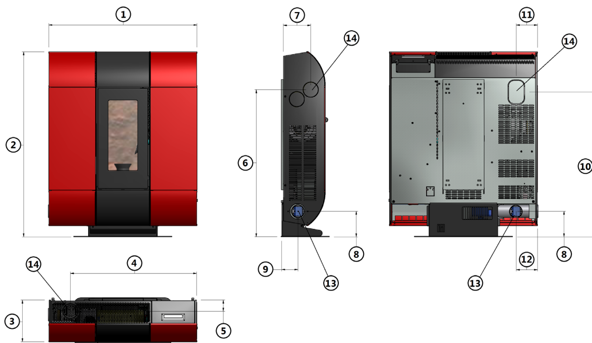
Fig. 11 - Allgemeine Abmessungen
