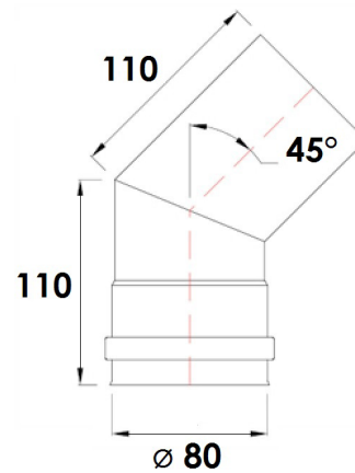
Fig. 13 - Krümmer 45°
