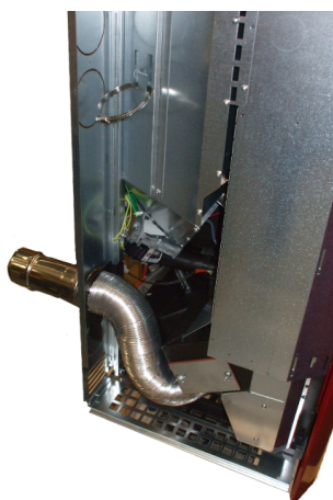
Fig. 47 - Positionierung der Rohre für hinteren Kanal
