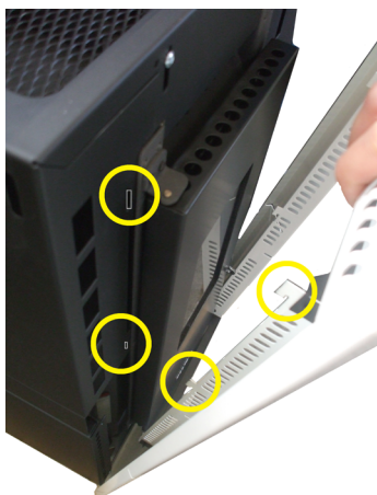
Fig. 36 - Montage Rahmen
