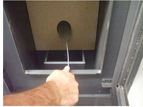
Fig. 59 - Reinigung mit Flaschenbürste
