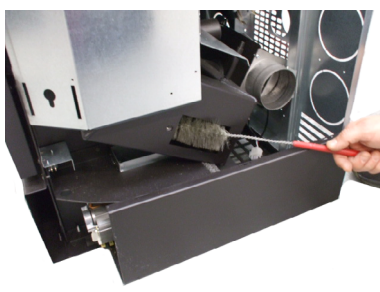
Fig. 80 - Reinigung mit Flaschenbürste 2
