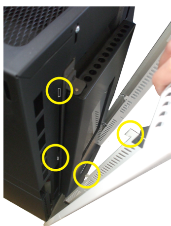
Fig. 22 - Montage Rahmen
