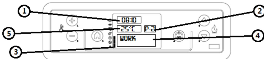
Fig. 51 - LC-Steuerdisplay
