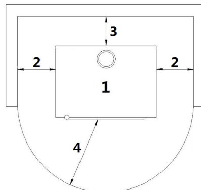
Fig. 21 - Allgemeine Installation
