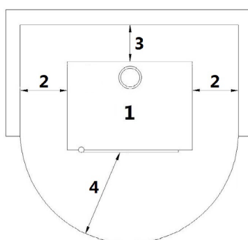
Fig. 19 - Allgemeine Installation
