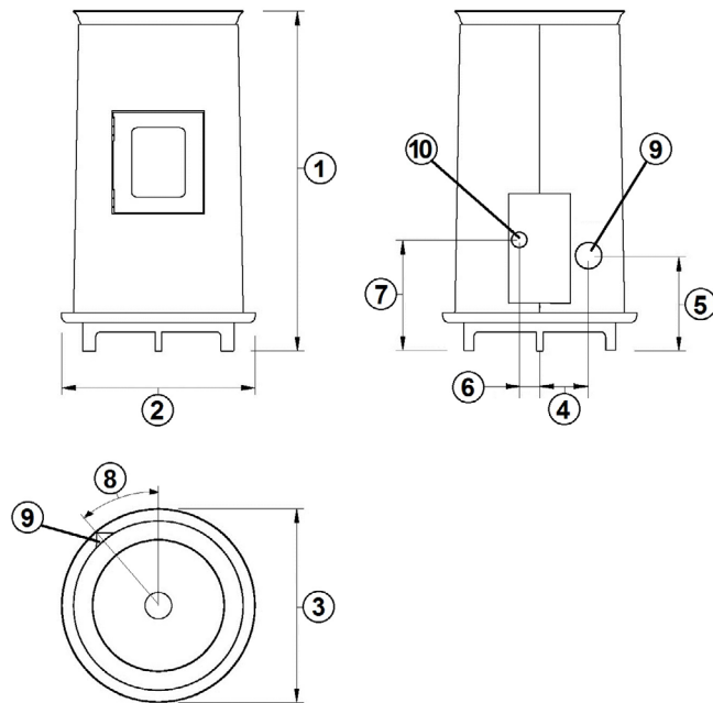
Fig. 17 - Allgemeine Abmessungen: Bistrot³
