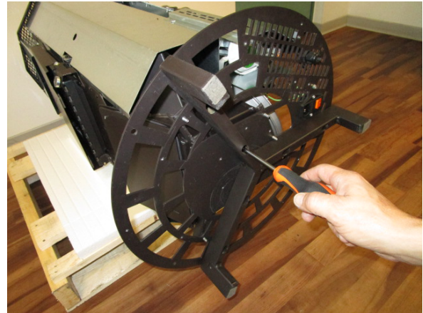
Fig. 46 - Die Schrauben entfernen
