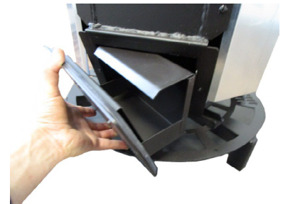
Fig. 95 - Kasten ausziehen
