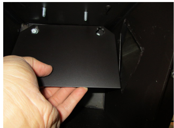
Fig. 97 - Rauchabweiser abnehmen
