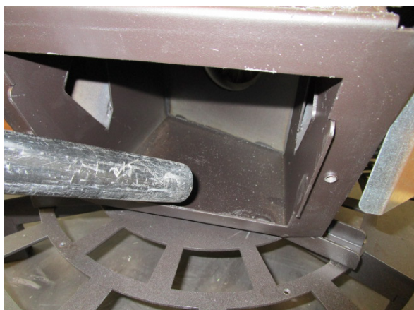
Fig. 98 - Asche absaugen
