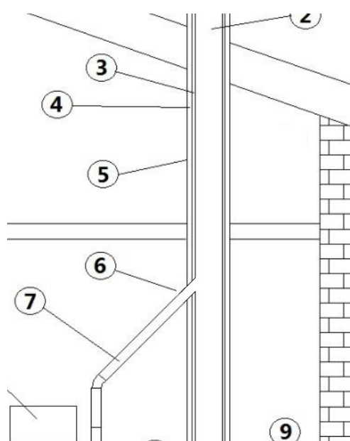
Fig. 5 - Bauteile Kamin
