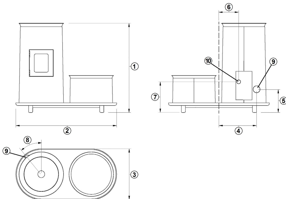
Fig. 18 - Allgemeine Abmessungen: Bistrot³ Lounge
