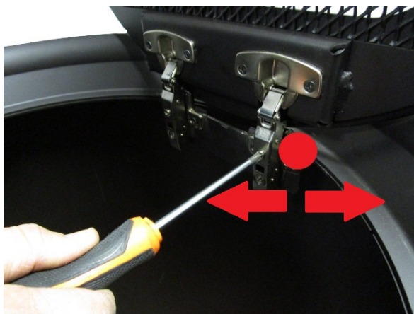
Fig. 61 - Regulierung der Zentrierung
