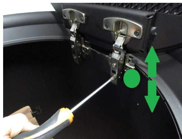
Fig. 62 - Regulierung der Höhe
