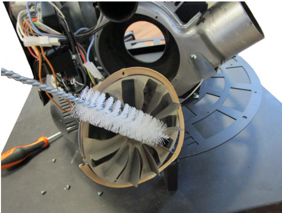
Fig. 104 - Reinigung Rauchgasansauggerät: Phase 1
