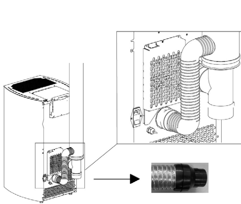
Fig. 9 - Flexibler Schlauch
