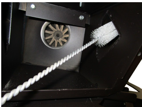
Fig. 100 - 1 - Reinigung mit Flaschenbürste
