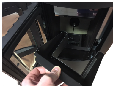
Fig. 87 - Aschenkasten entnehmen
