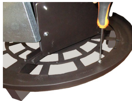
Fig. 38 - Schrauben befestigen
