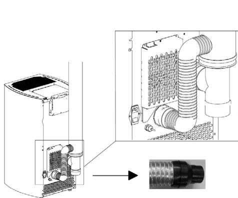
Fig. 9 - Flexibele buis
