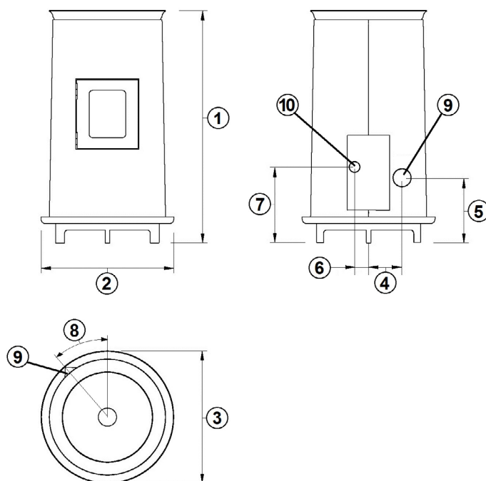
Fig. 17 - Algemene afmetingen: Bistrot 3
