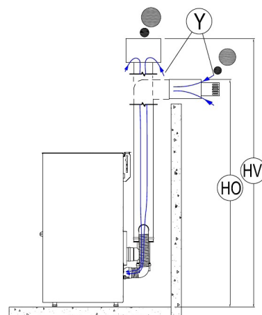
Fig. 11 - Verbindingen schoorsteenpijp
