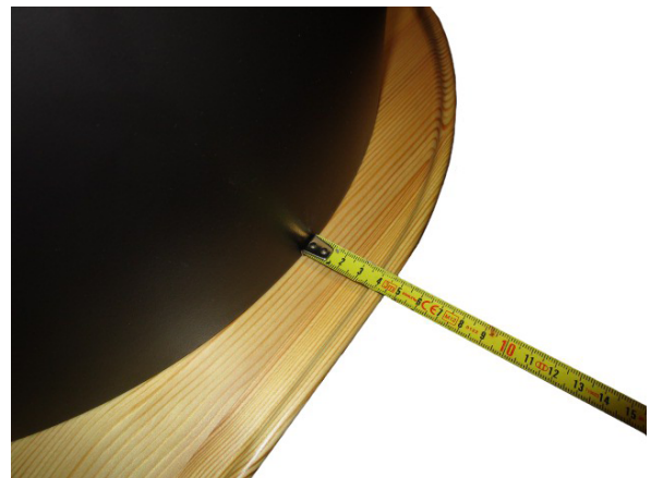
Fig. 58 - Correcte positionering
