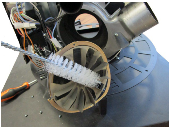
Fig. 104 - Reiniging rookgassenafzuiger: fase 1
