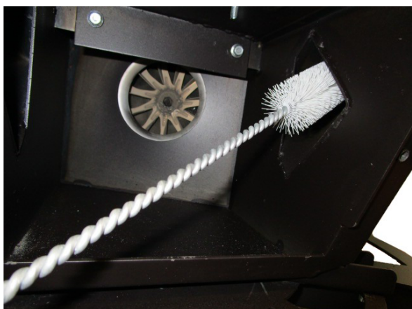
Fig. 100 - Reiniging met pijpenwisser 1
