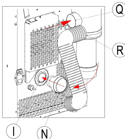
Fig. 10 - Verbindingen
