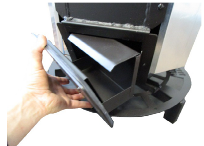
Fig. 95 - Verwijdering van de lade
