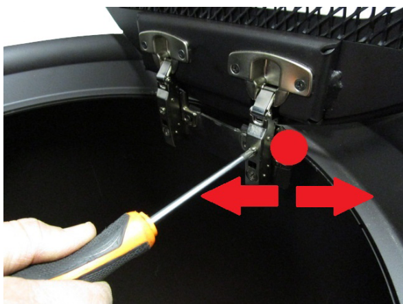
Fig. 61 - Regeling centrering
