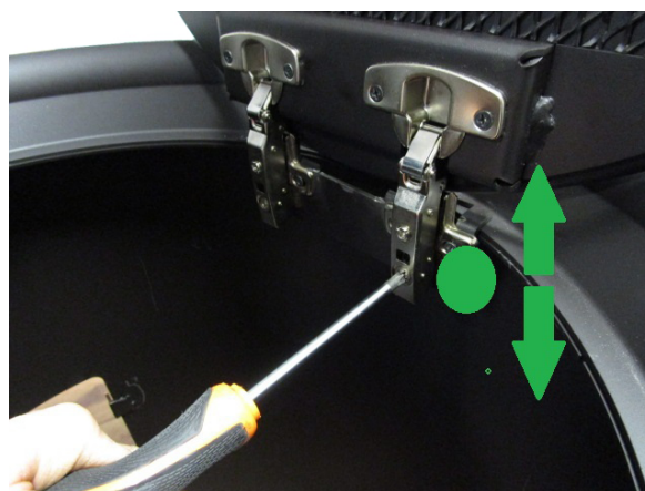
Fig. 62 - Regeling hoogte
