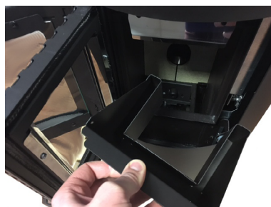
Fig. 87 - Verwijdering aslade
