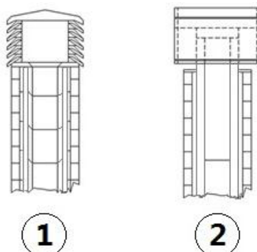
Fig. 4 - Windbestendige schoorsteenpotten
