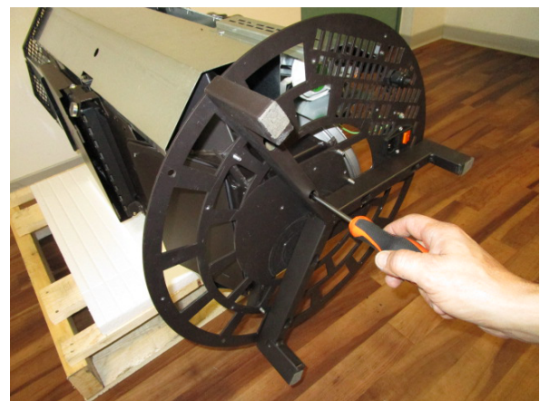
Fig. 46 - Verwijder de schroeven
