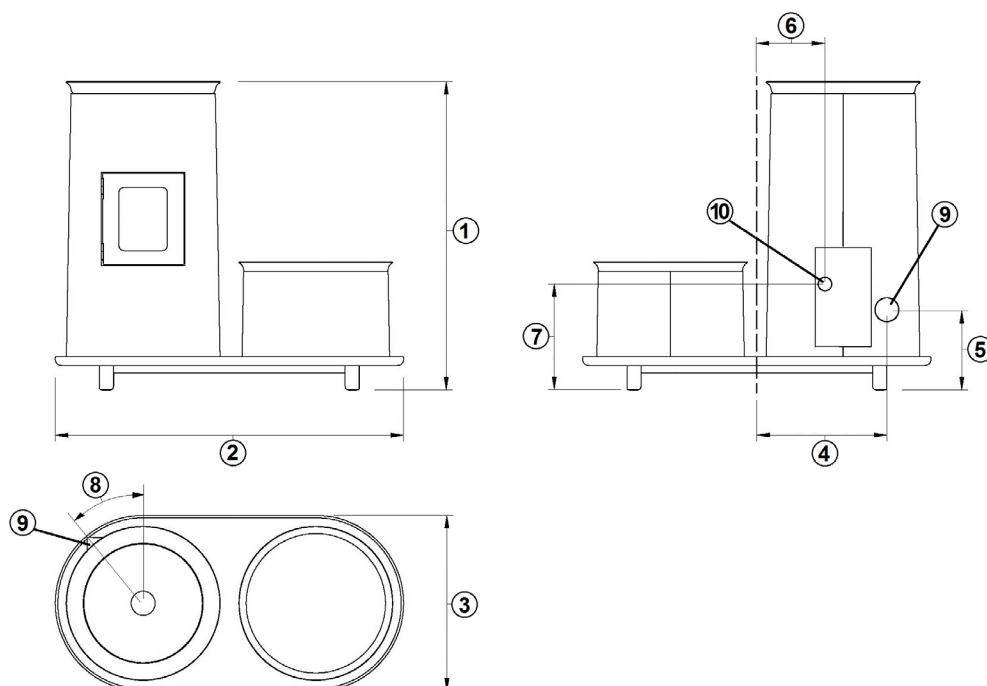
Fig. 18 - Algemene afmetingen: Bistrot 3 Lounge
