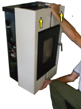
Fig. 22 - Retirez les côtés: phase 1
