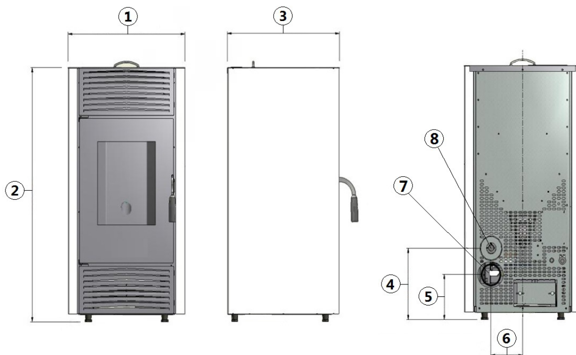
Fig. 11 - Dimensions générales
