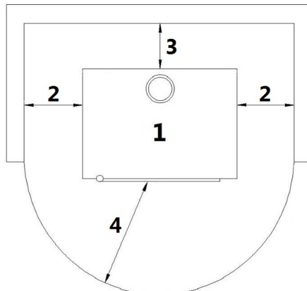
Fig. 12 - Installation générale
