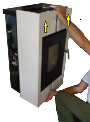
Fig. 22 - Estrarre fianchi: fase 1
