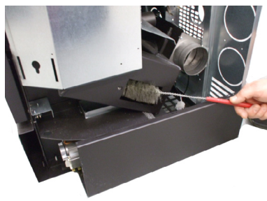
Fig. 80 - Reiniging met flessenwisser 2
