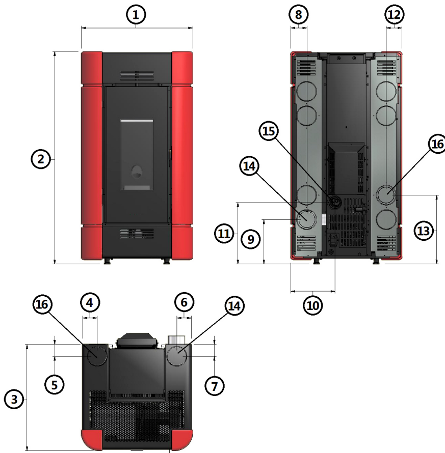
Fig. 16 - Algemene afmetingen: Sire³ Plus
