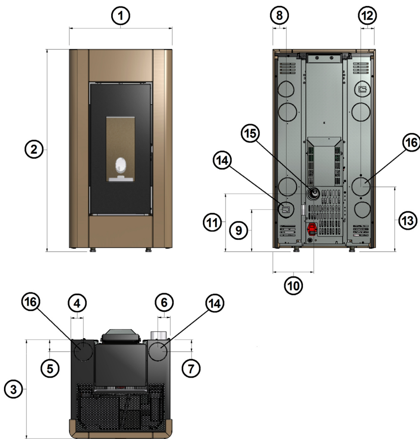
Fig. 19 - Algemene afmetingen: Prince 3 / Prince 3 Plus
