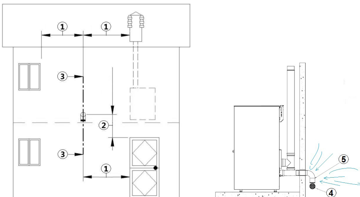
Fig. 8 - Luchtinlaat voor installatie met hermetisch gesloten kamer
