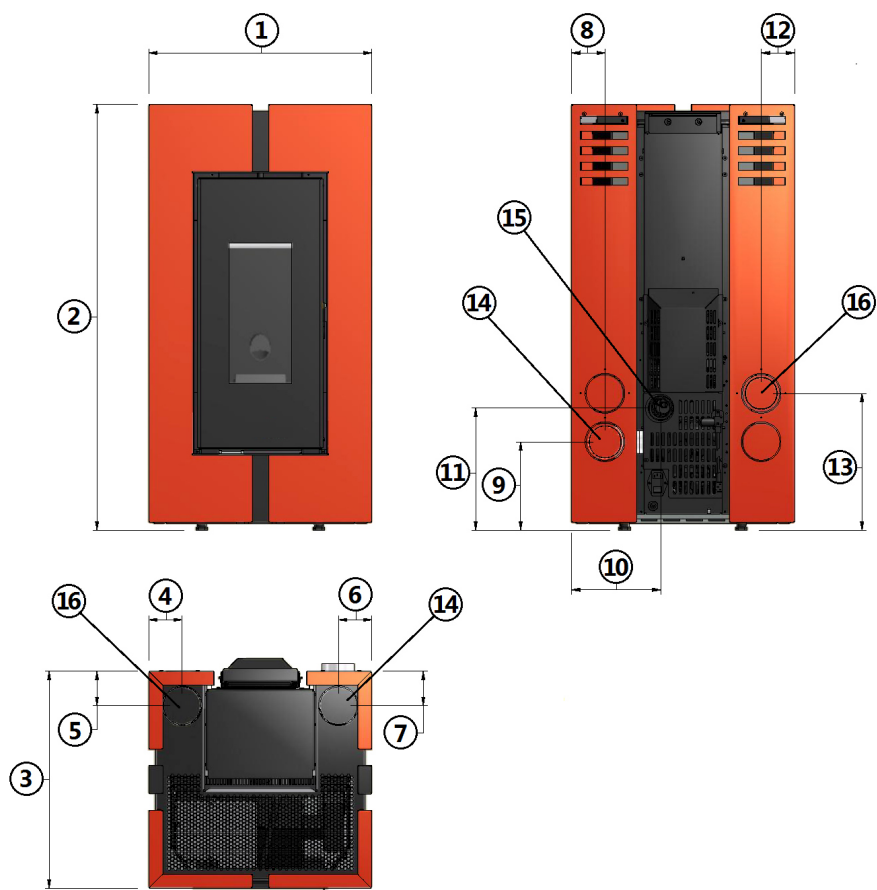
Fig. 17 - Algemene afmetingen: Doge 3 Plus
