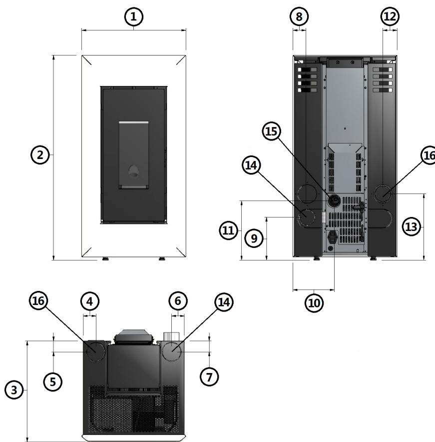
Fig. 15 - Algemene afmetingen: Vega / Trend
