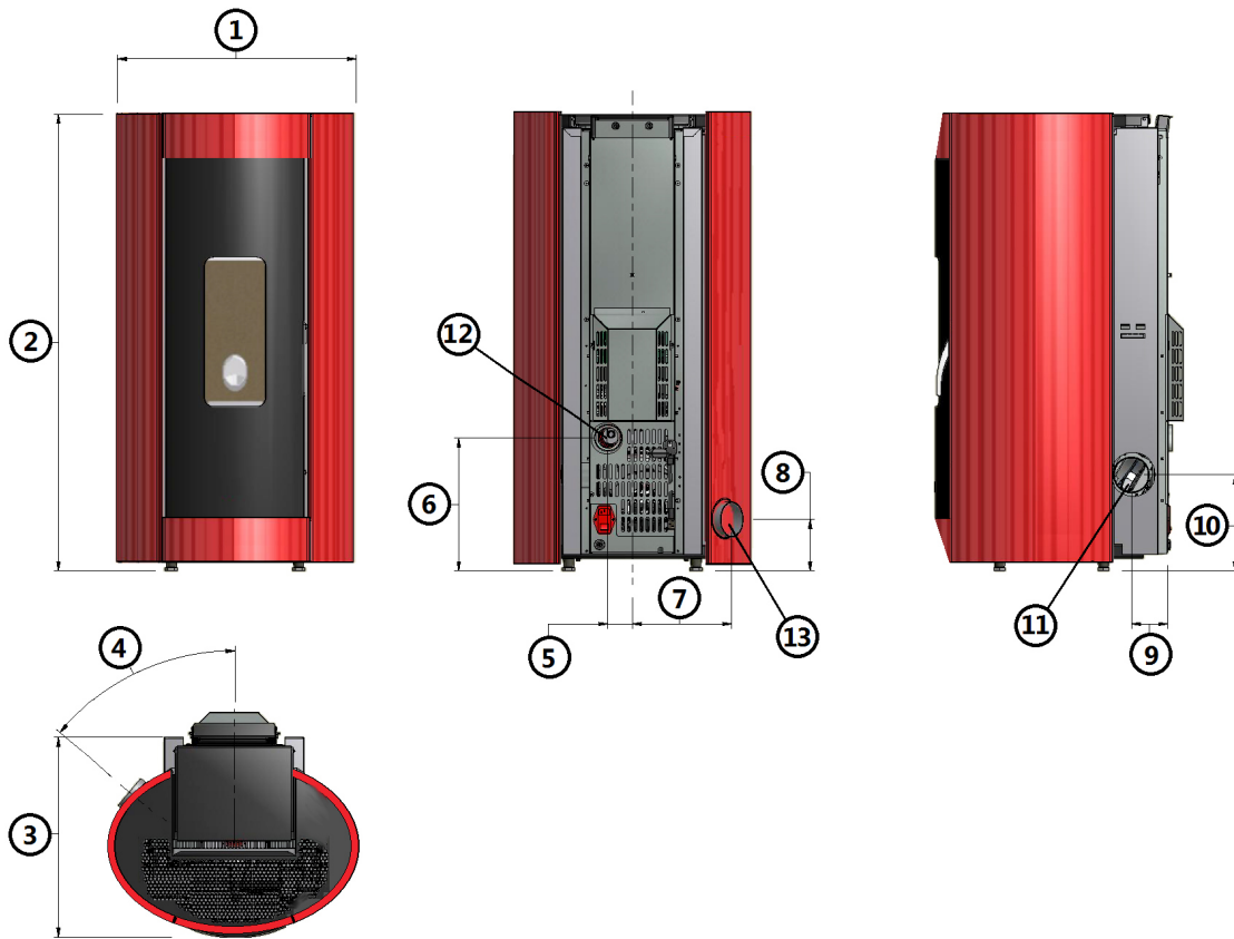
Fig. 20 - Algemene afmetingen: Elise 3 Plus
