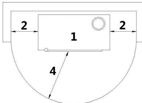
Fig. 18 - Wandinstallation
