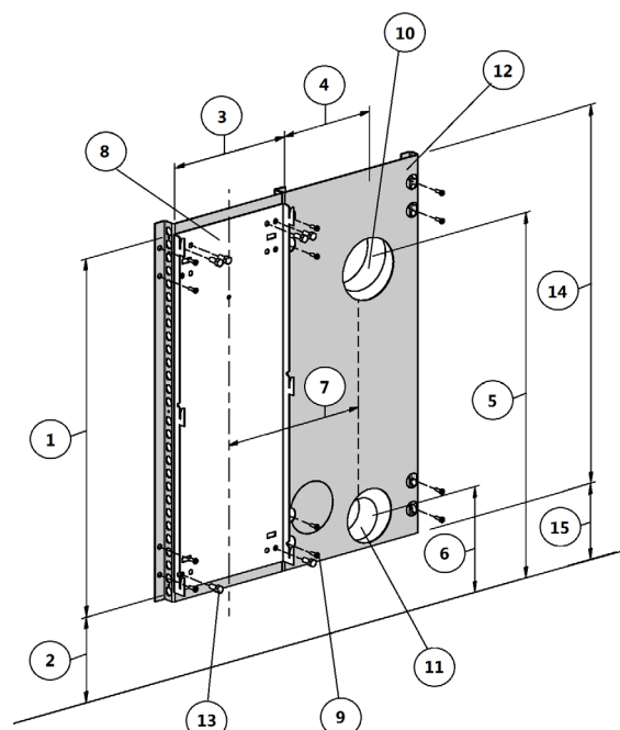
Fig. 20 - Befestigung an einer brennbaren Wand
