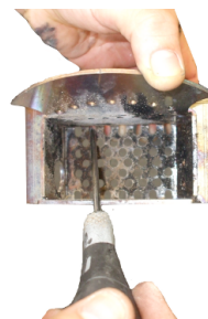
Fig. 29 - Reinigung Brennschale
