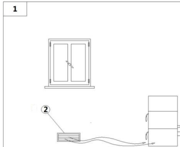
Fig. 6 - Direkte Luftzufuhr
