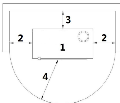
Fig. 15 - Allgemeine installation mit Sockel
