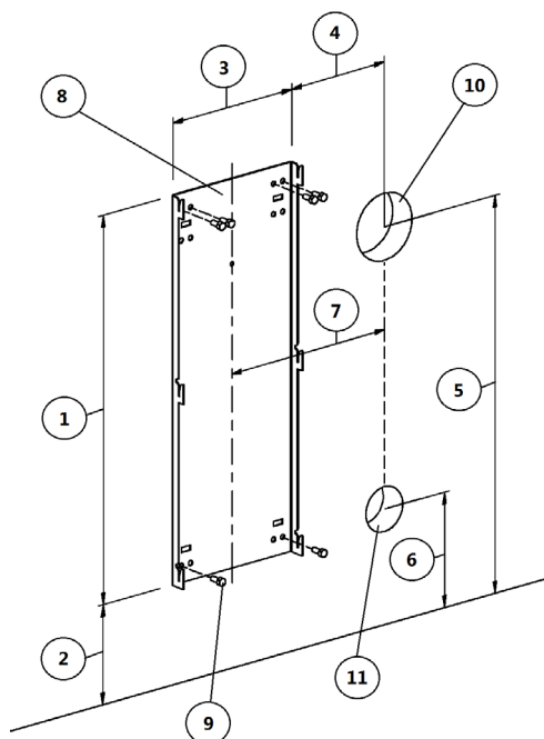
Fig. 19 - Befestigung an einer nicht brennbaren Wand
